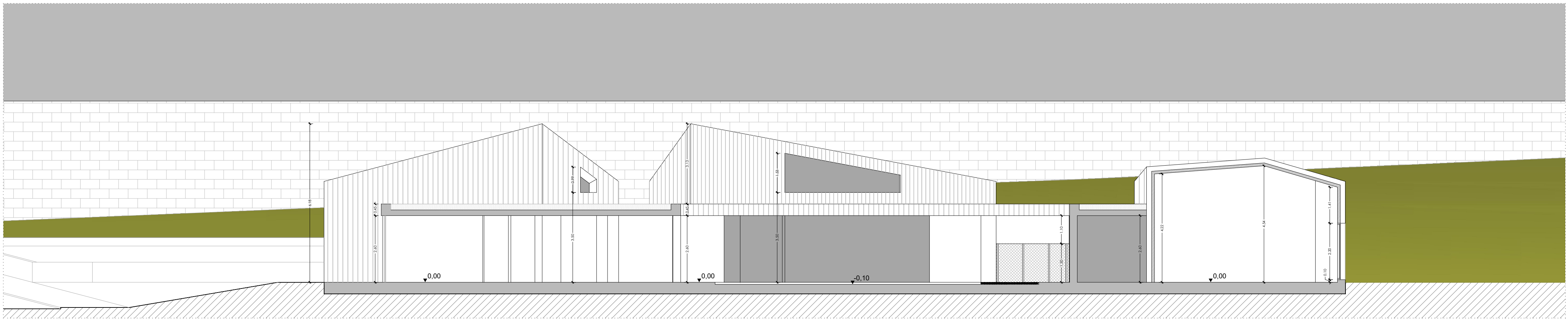
SECCIÓN C C'
