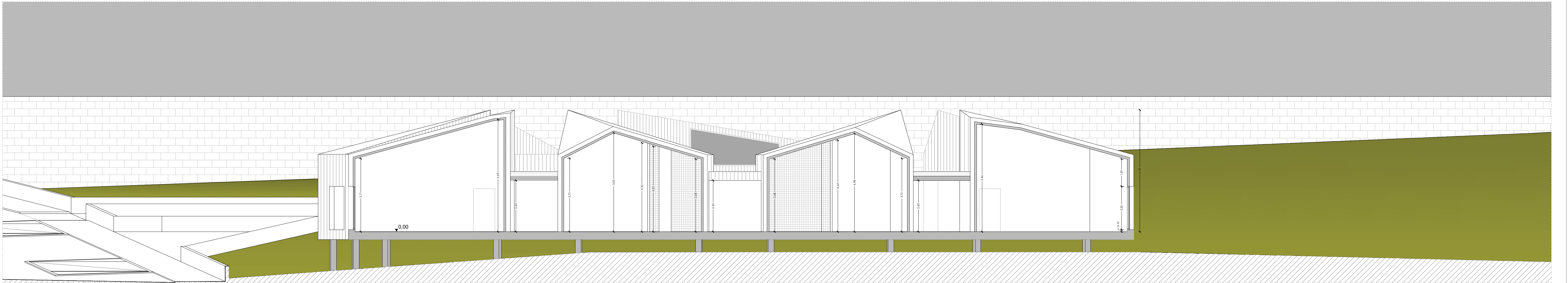
SECCIÓN A A'
