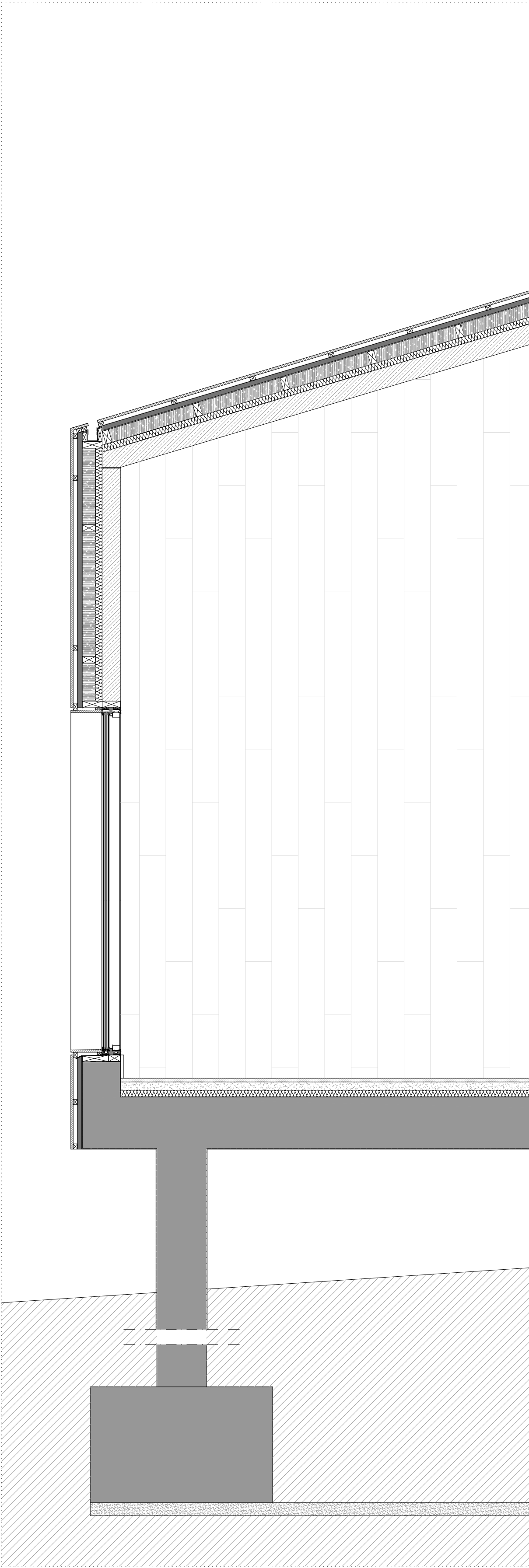
Sección constructiva C 1
