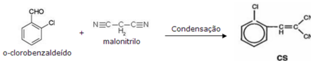
Figura 7 – Síntese do gás CS por condensação do o-clorobenzaldeído com o malonitrilo (A) [3]
