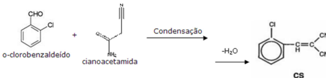
Figura 8 – Síntese do gás CS por condensação do o-clorobenzaldeído com cianoacetamida (B) [3]
