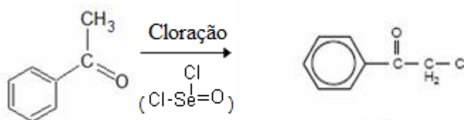
Figura 10 – Síntese do gás CN [3]
