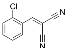
Figura 6 – Fórmula de Estrutura do CS [8]
