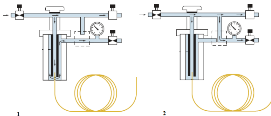
Figura 17 – (1) – Injeção em modo split (2) – Injeção em modo splitless [26]
