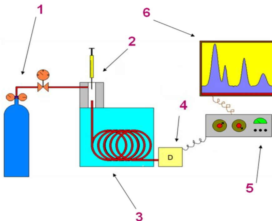
Figura 16 – Esquema de uma montagem de GC [20]
