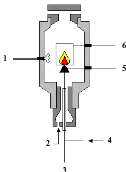
Figura 18 – Ilustração de um detetor FID [33]
