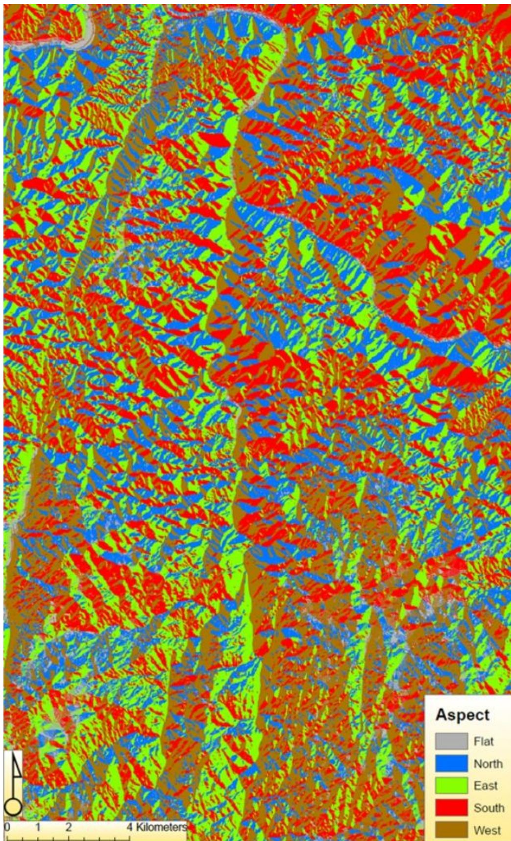
Figura 22. Orientação das encostas em nossa área de estudo. Este mapa foi realizado no software ArcView 9 usando um DTM com uma resolução de 10 metros fornecido pelo Instituto Geográfico Português (IGEO - www.igeo.pt ).
