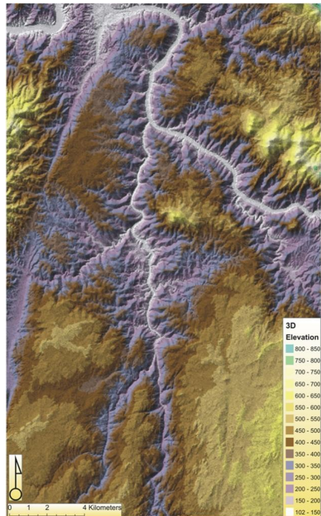
Figura 2. Altitude na nossa área de estudo, os últimos 17 kms. do rio Côa e sua confluência com o Douro.
