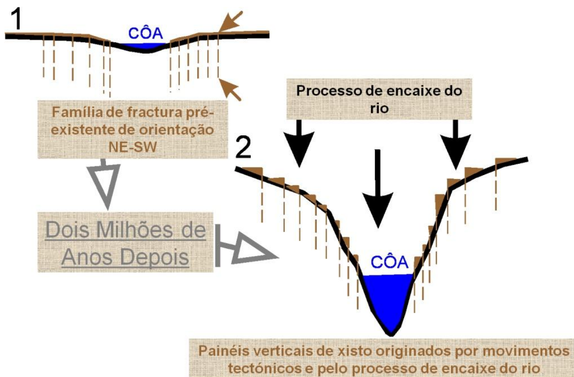
Figura 3. Ilustração esquemática do processo de encaixe do Côa.
