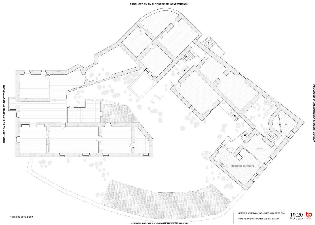
Figura 37 - Planta da Casa da Pequenina Piso_1
