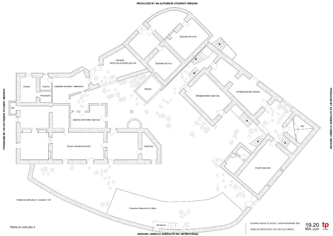
Figura 36 - Planta da Casa da Pequenina Piso_0
