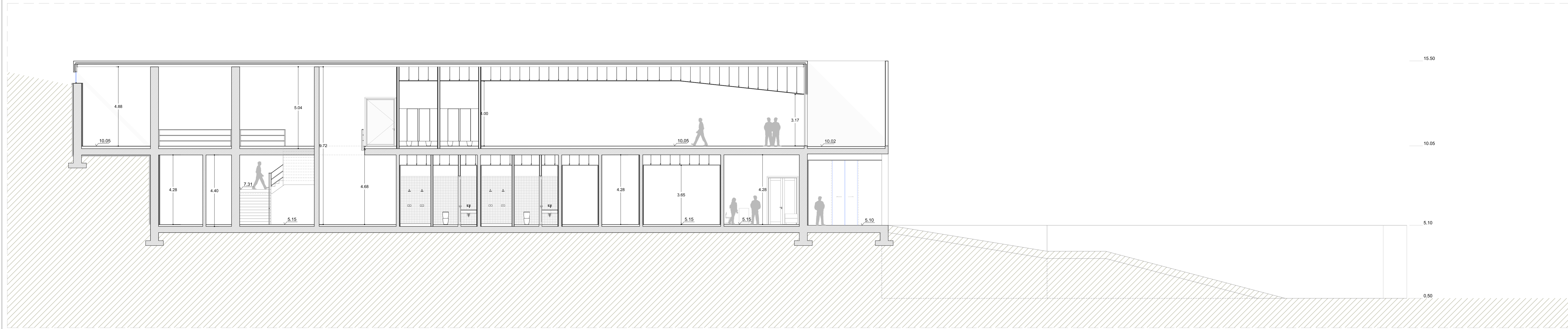
CORTE/ALÇADO 1
