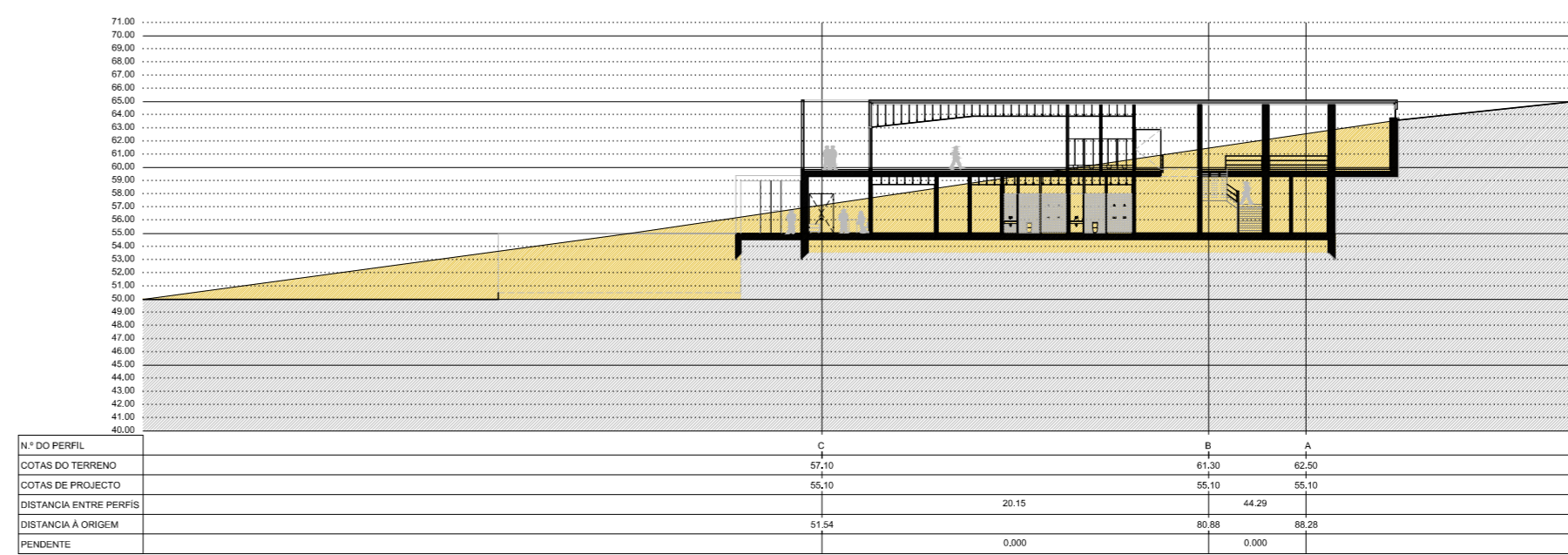
PERFIL TRANSVERSAL FF
