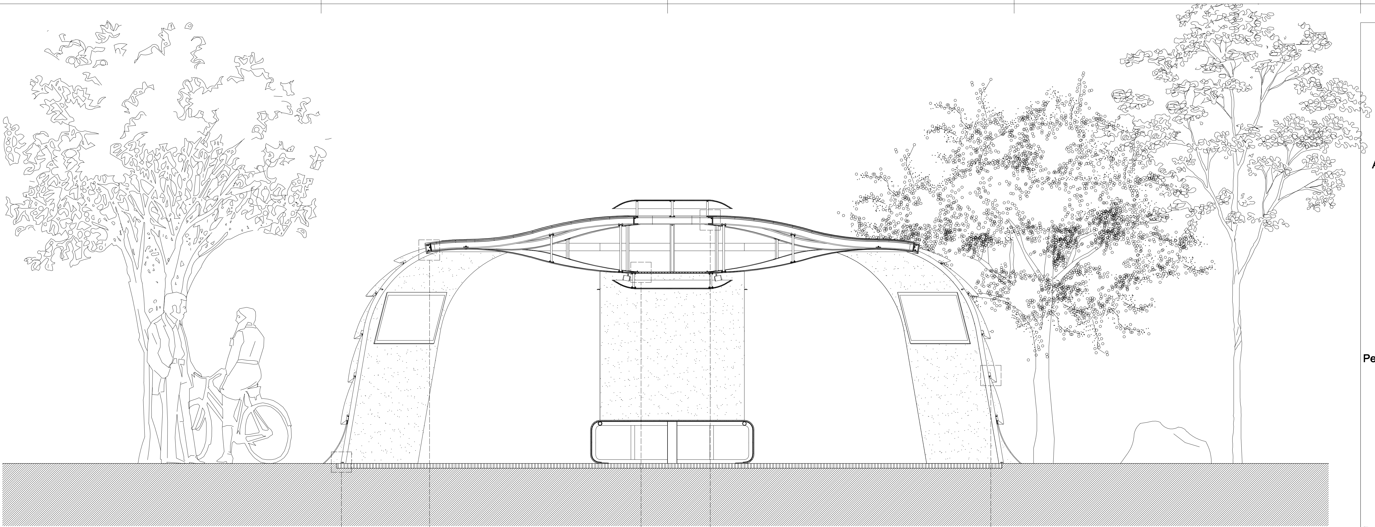
Corte C
