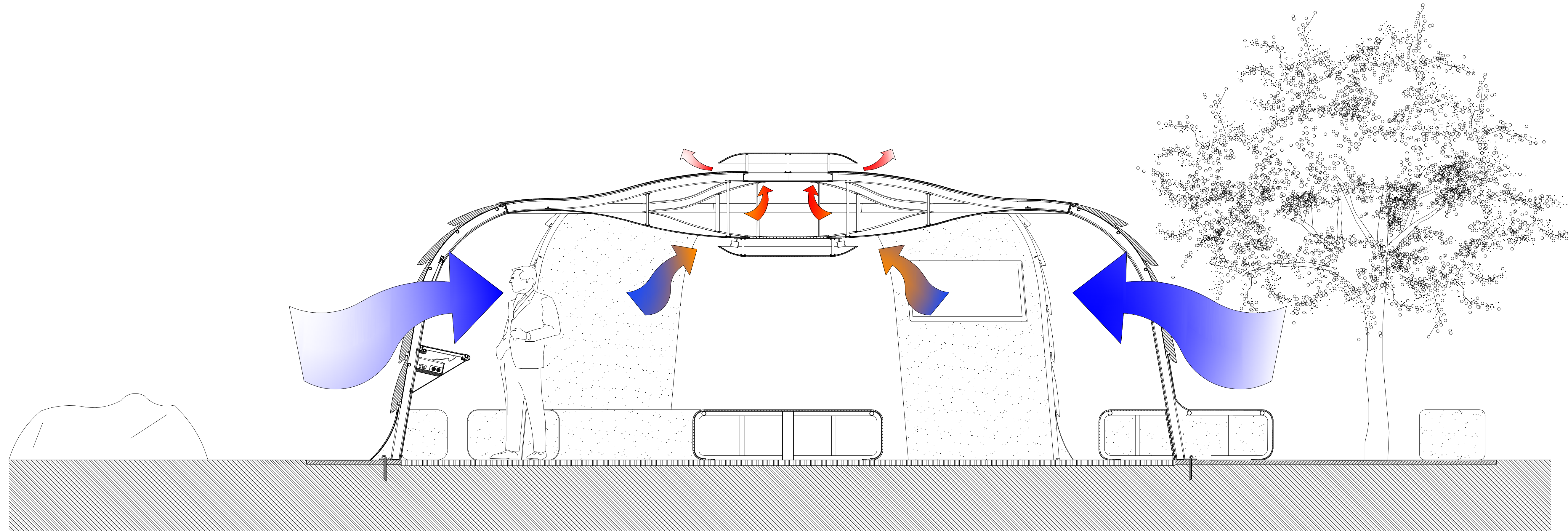
Corte B
