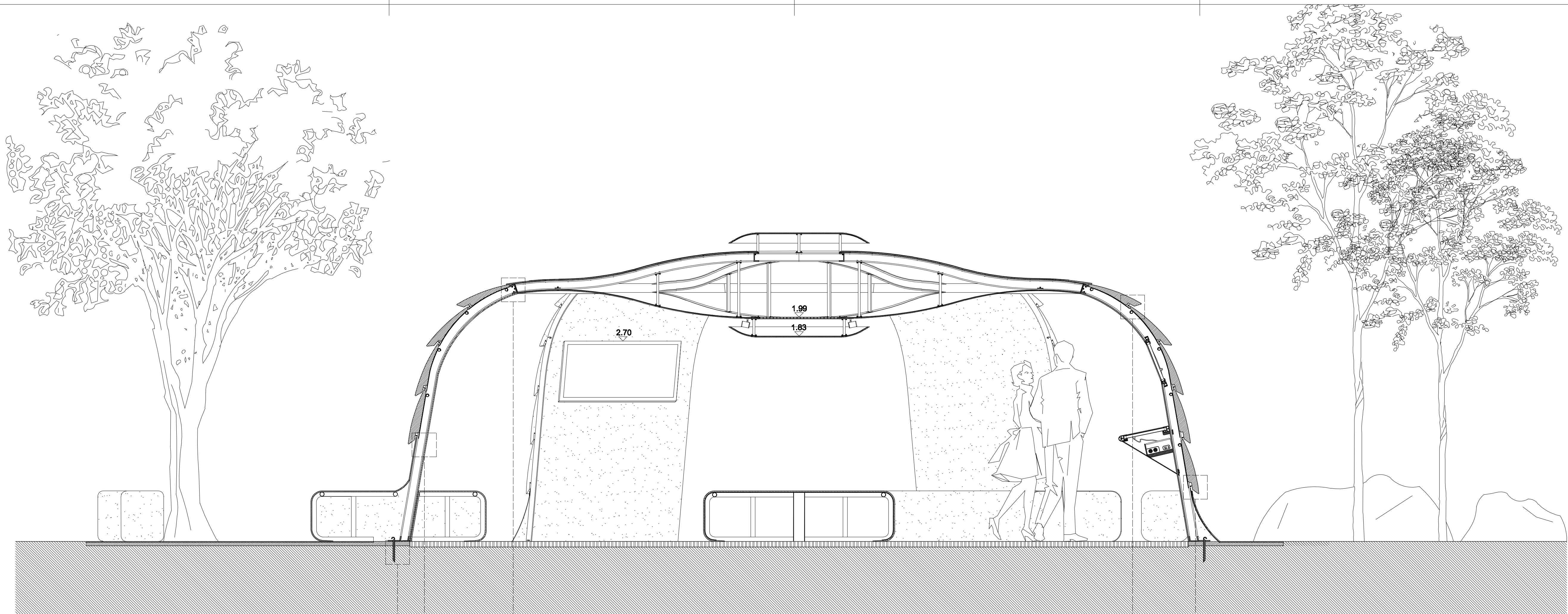
Corte A
