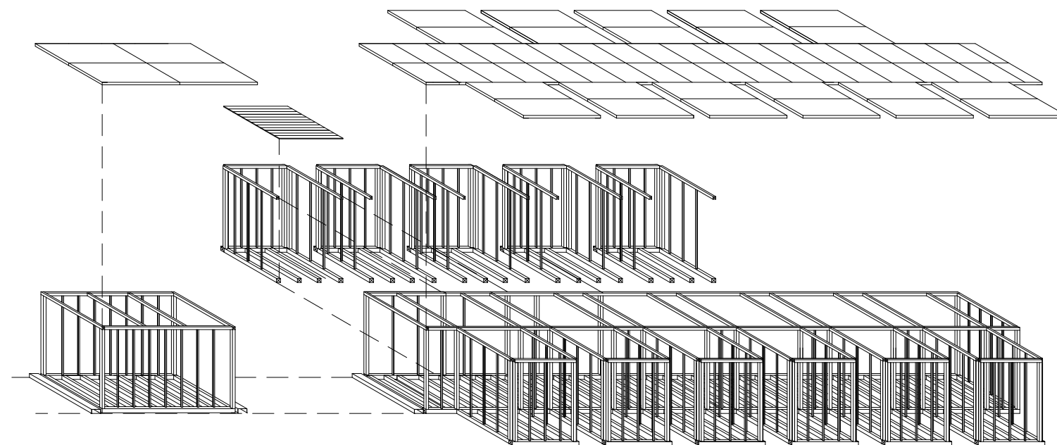
axonometria explodida com sistema construtivo de madeira
