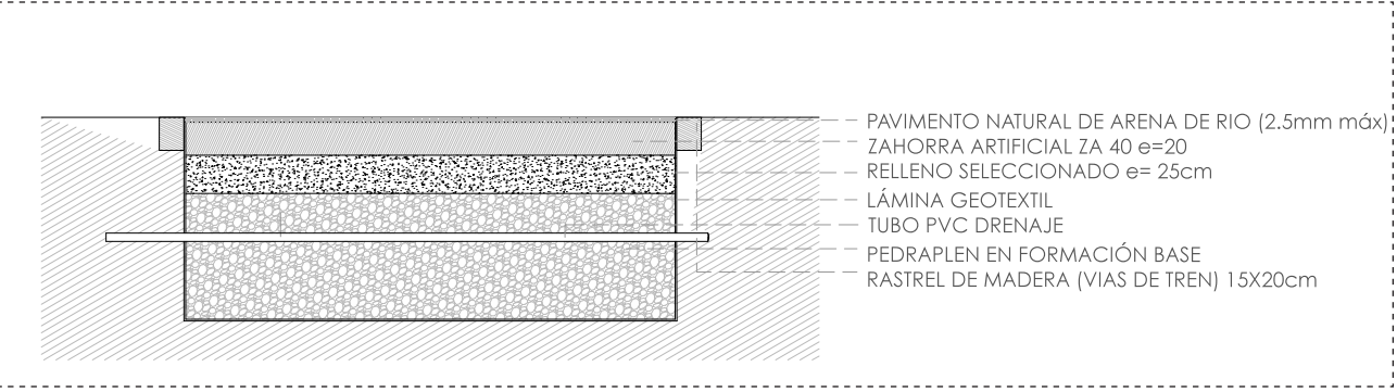
Corte Sendero 3, Esc: 1/50
