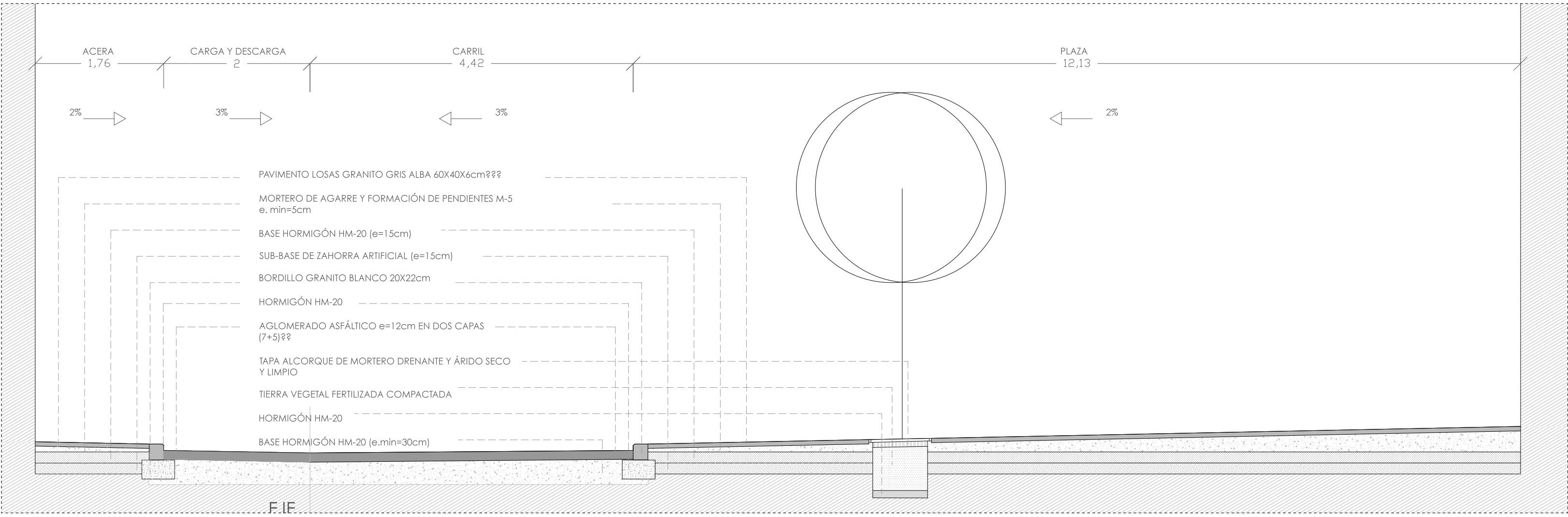
Corte B, Esc: 1/50
