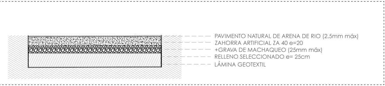
Corte Sendero 2, Esc: 1/50
