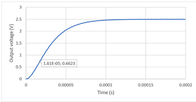
Fig. 12. Step response.
