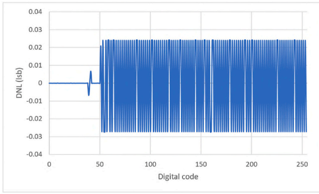
Fig. 11. DNL.
