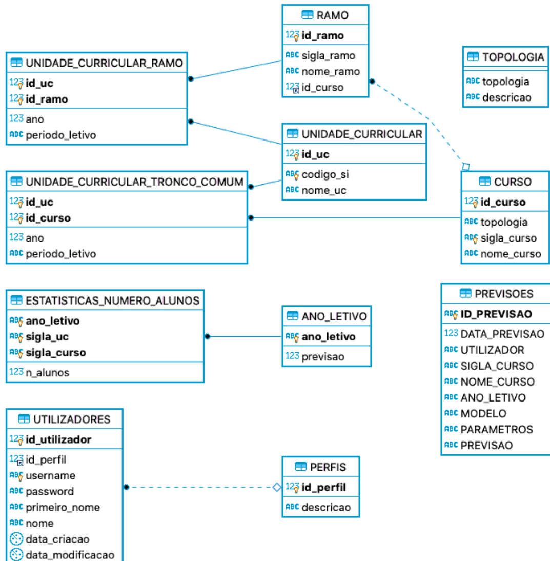
Figura 2.1.4 - Modelo relacional da base de dados
