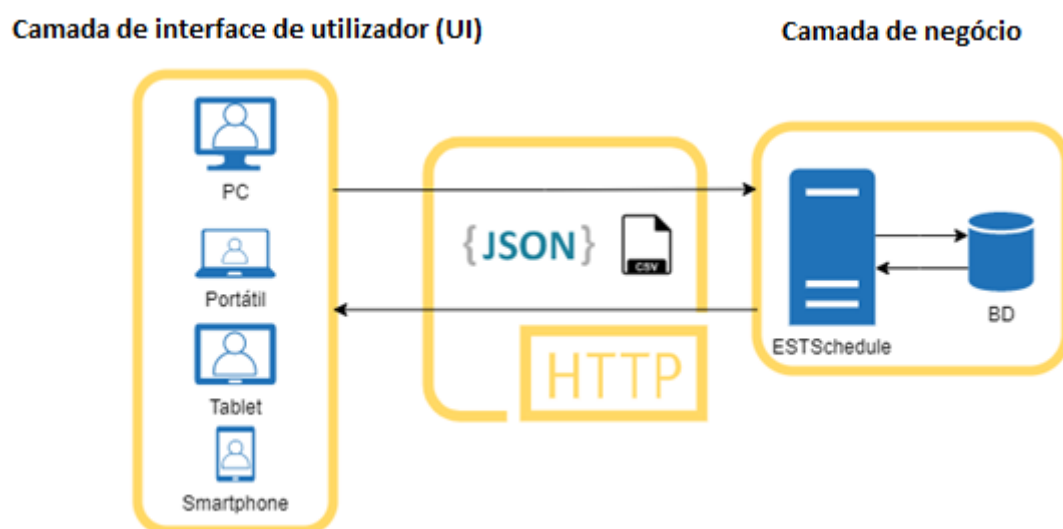
Figura 2.1.1 - Desenho de alto nível da arquitetura do projeto ESTSchedule
