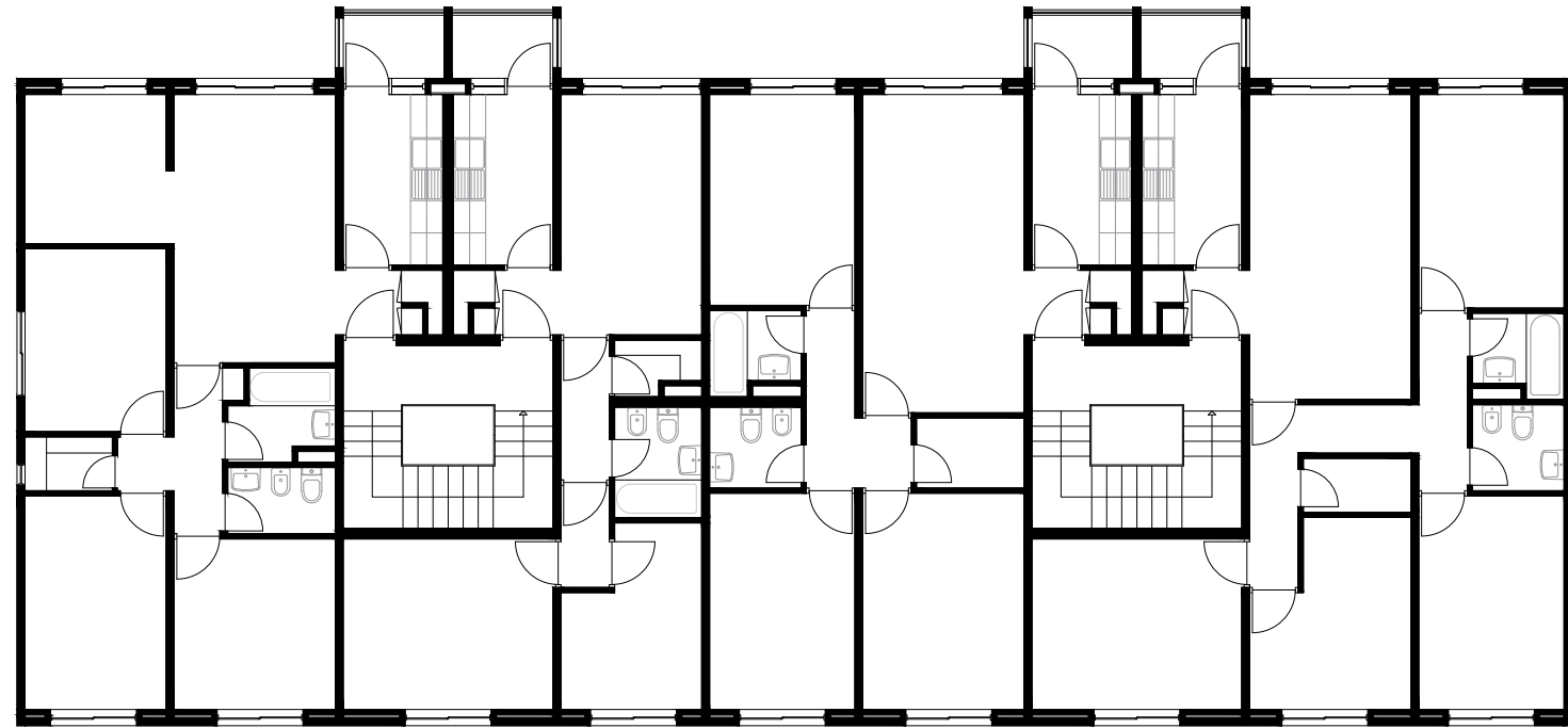
PISO TIPO
