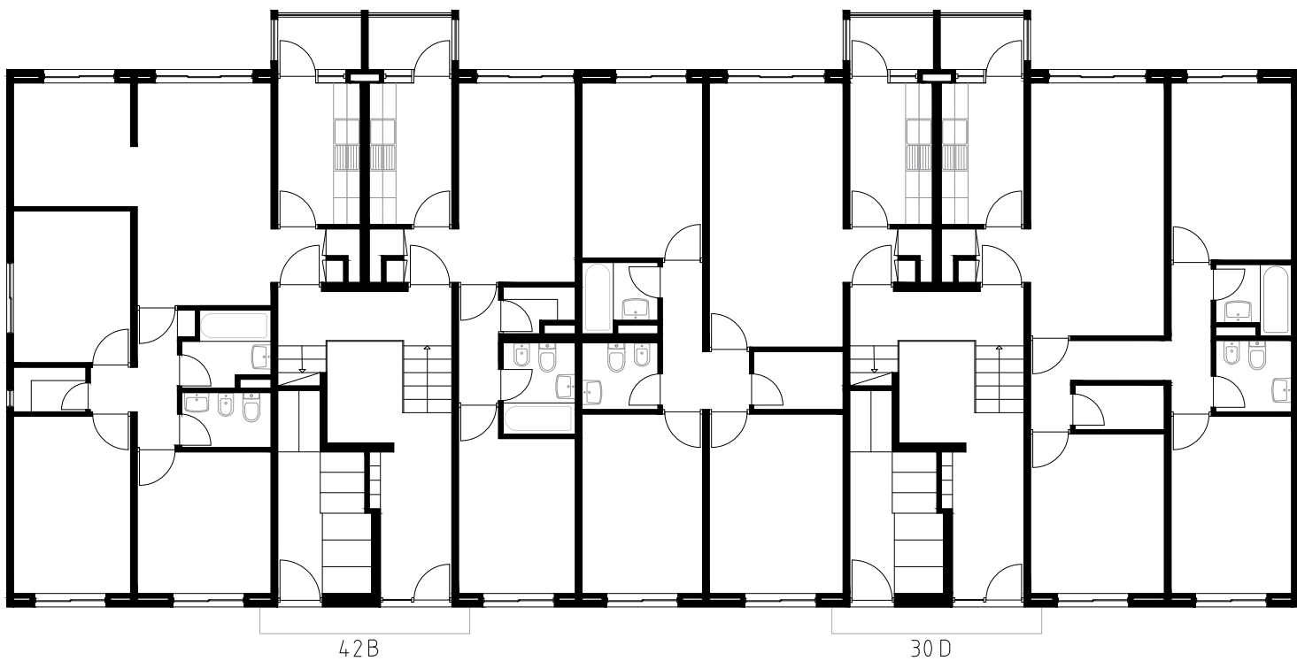
PISO TÉRREO
