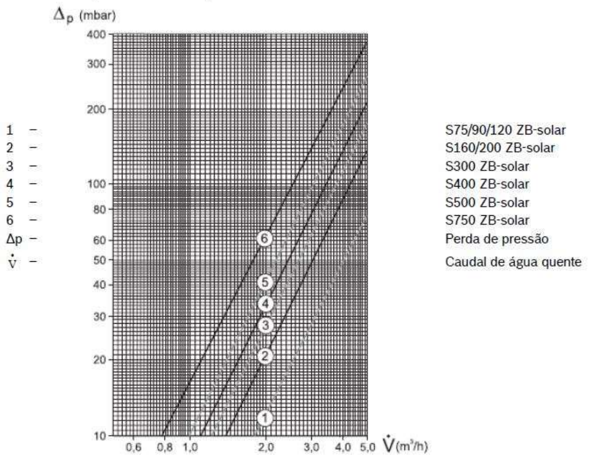
Anexo 5. Gráfica de perda de carga do Depóstip S750 ZB-Solar
