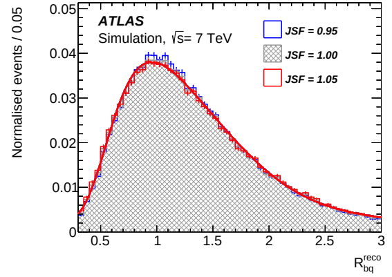
(d) R_{bq}^{\text{reco}} , at least two b -tagged jets
