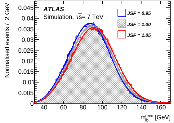
(d) m_{\ell b}^{\text{reco}} , exactly two b -tagged jets
