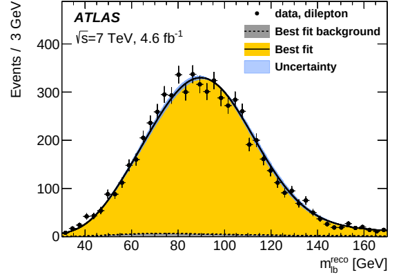
(d) m_{lb}^{\text{reco}}, \text{dilepton}
