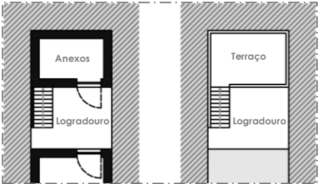
Fig. 308 – Terraço, tipologia 2 Esc:1/200
