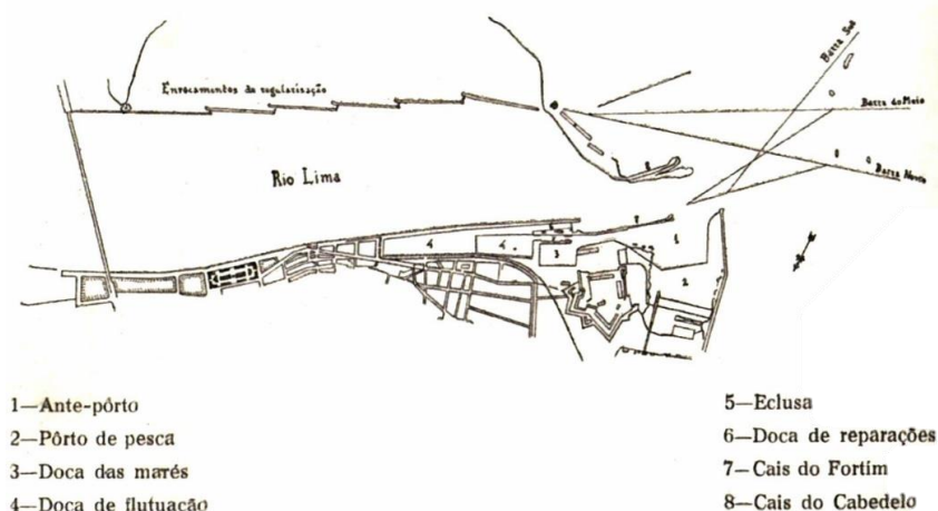
Fig.23 - Construção do atual porto de Viana
