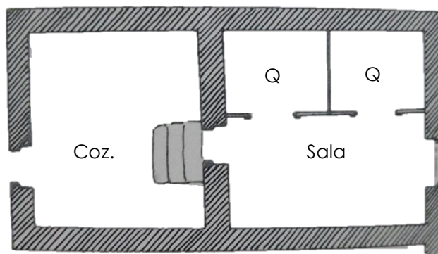
Fig.16 – Planta de casa tipo s/escala
