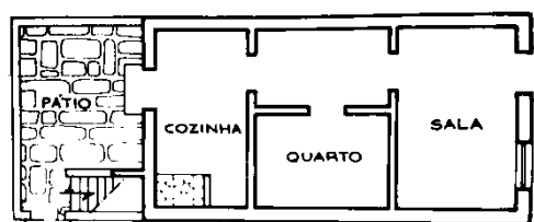
Fig.9 – Planta de uma habitação típica da região do Algarve
