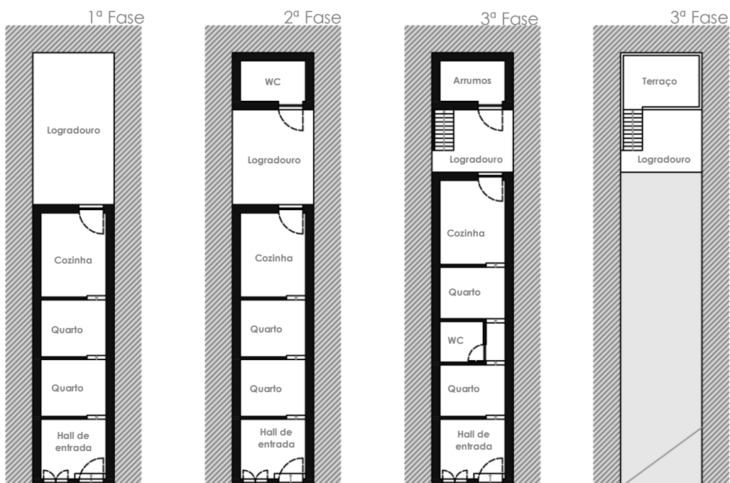
Fig.41 - Exemplo das três fases de evolução Esc: 1/200
