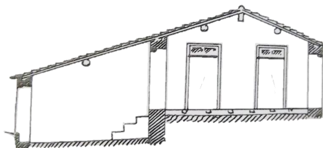
Fig.17 – Corte de casa tipo s/escala
