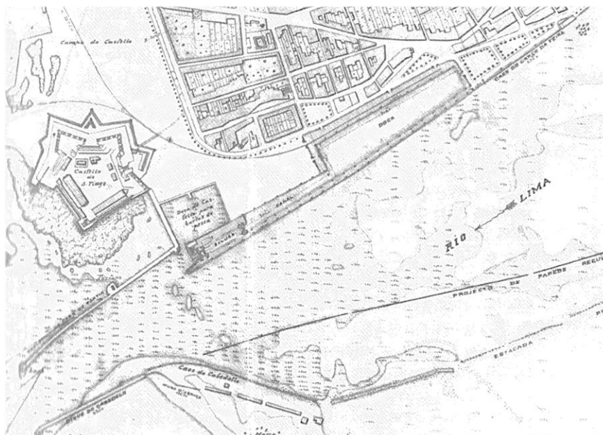
Fig.22 - Planta do porto, após as primeiras obras
