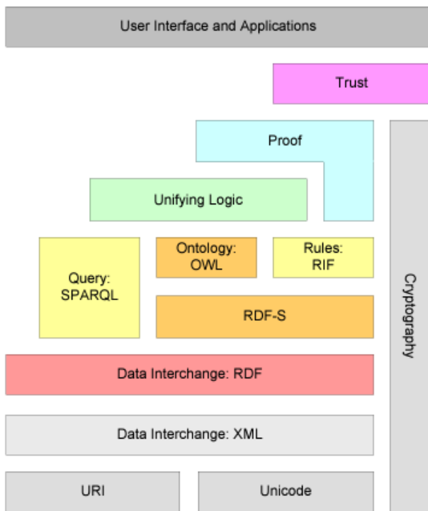
Figure 2 – The semantic webstack (Berners-Lee,2009,p.14)
