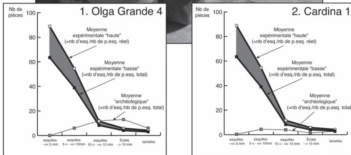
FIG. 5.1.4.1-2 – Reconstitution expérimentale du schéma de production sur nucléus bipolaires sur enclume et quantification du nombre moyen d'esquilles produites par classes de taille. À noter : le « nb de pièces esquillées total » = la totalité des pièces esquillées sans remontage les unes avec les autres ; le « nb de pièces esquillées réel » = le nombre de pièces réel qui a été débité (donc avec remontage ; en effet, au cours du débitage, il peut y avoir fracturation d'un artefact en deux ce qui conduit à deux pièces esquillées au lieu d'une, d'où un décalage entre « nb total » et « nb réel »). La moyenne archéologique correspond aux quantifications effectuées pour les sites. (Cliché L. Klaric).
