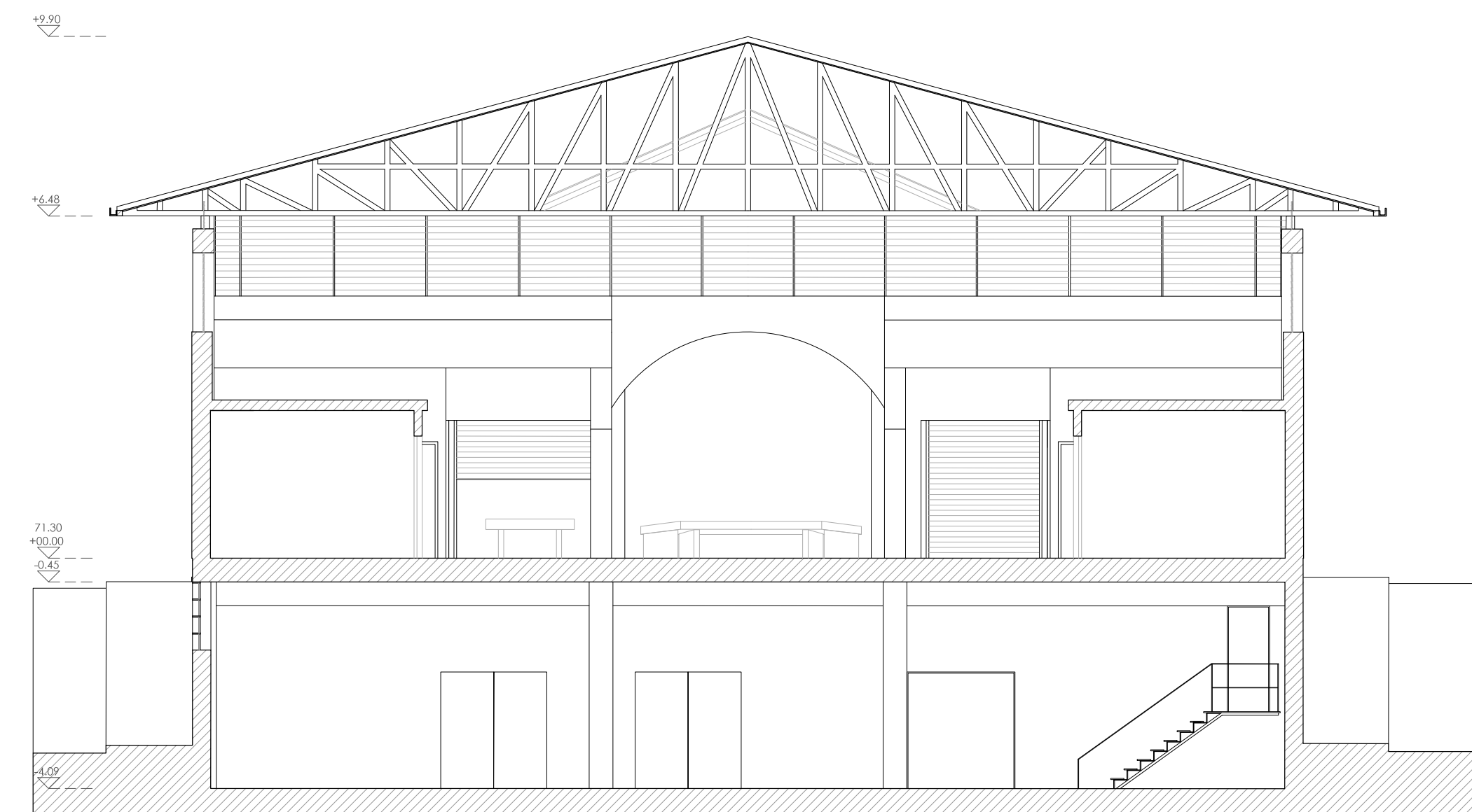
Corte B
