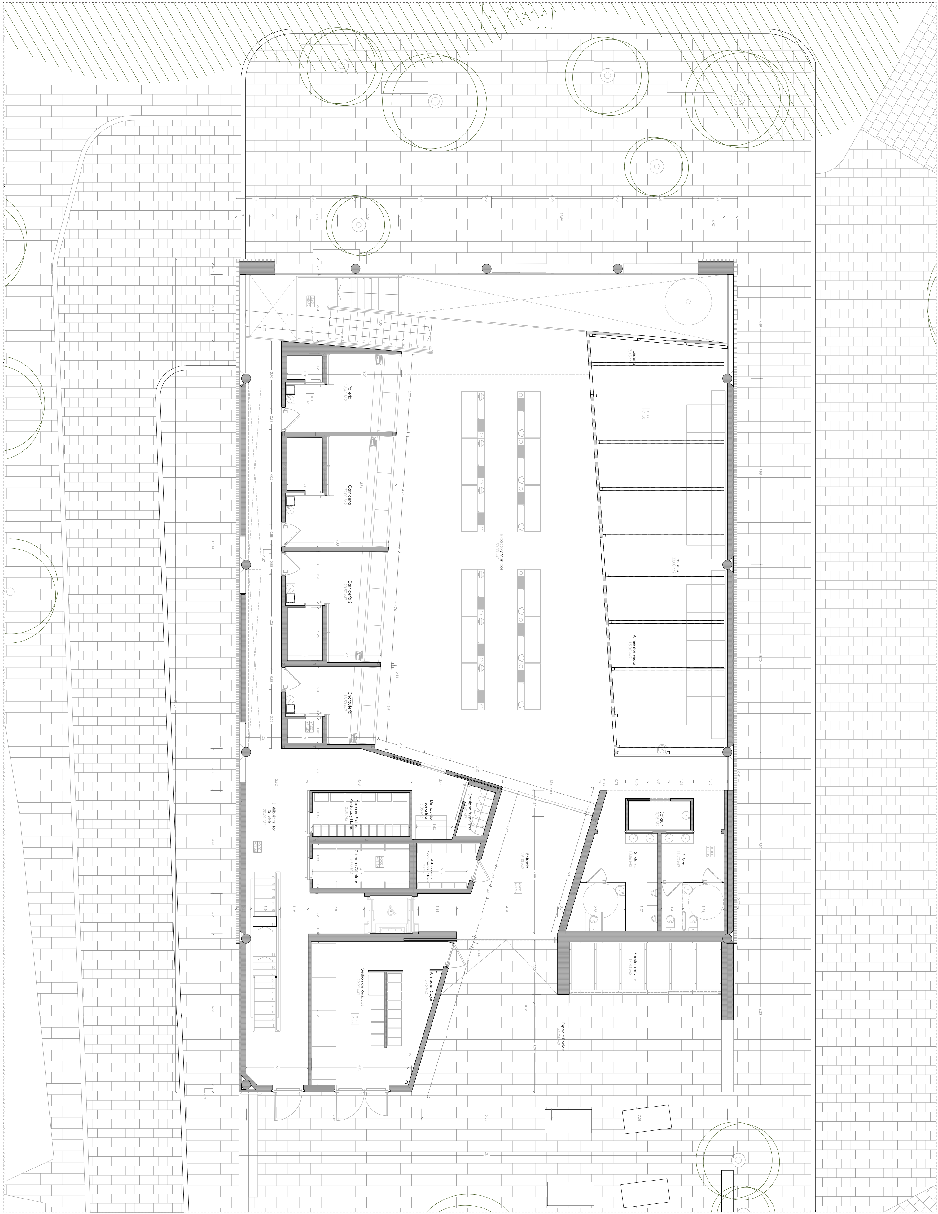
Planta piso 0, cota +0,00
