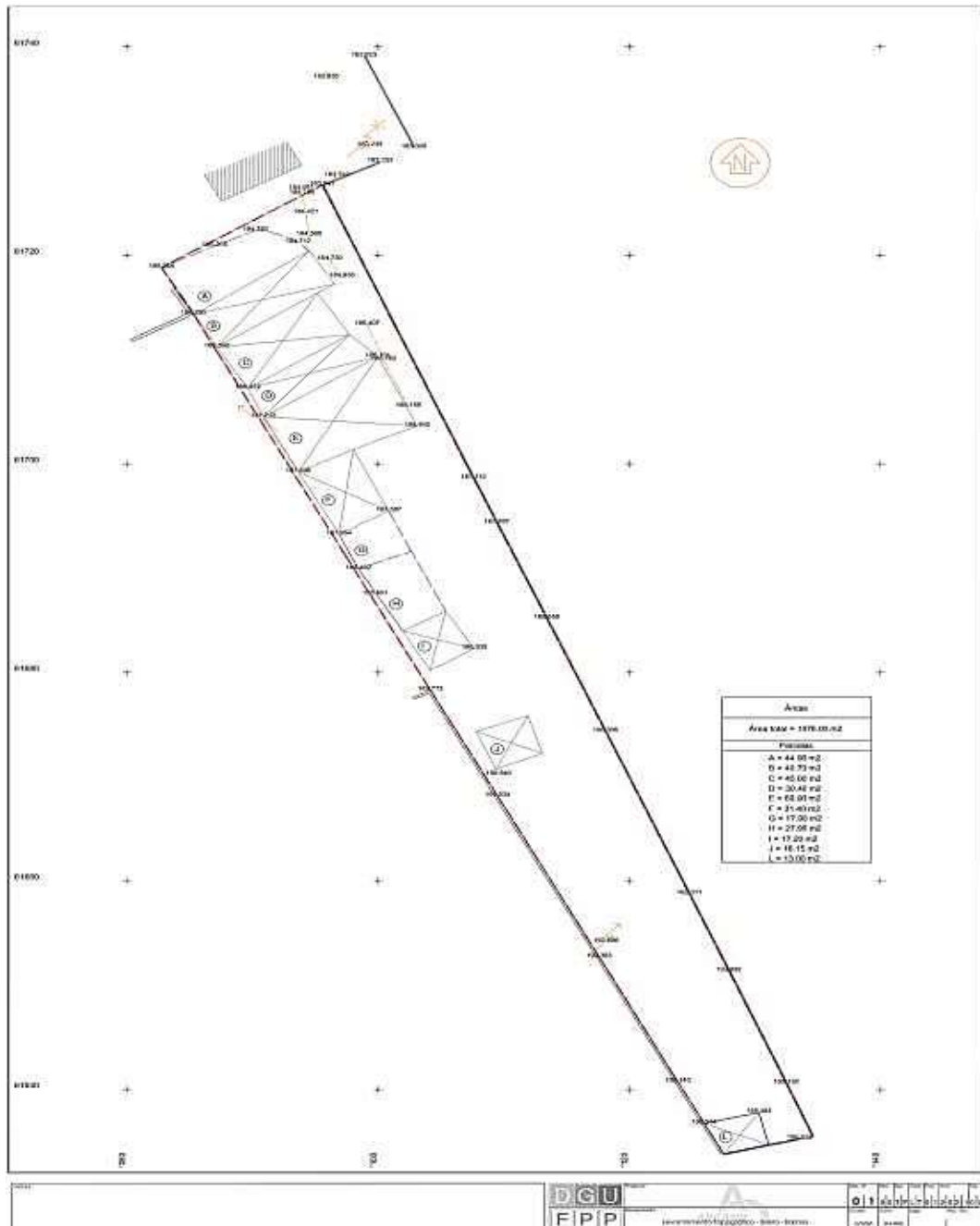
Figura 5 - Mapa Topográfico da zona superior do Bairro São Vicente de Paulo (Zona de cultivo, de acesso aos animais e de arrumos)
