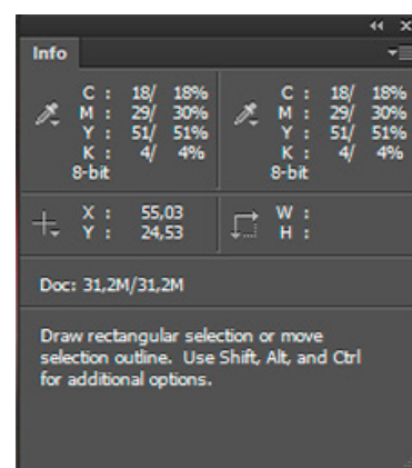
FIG.01 - Janela Info
