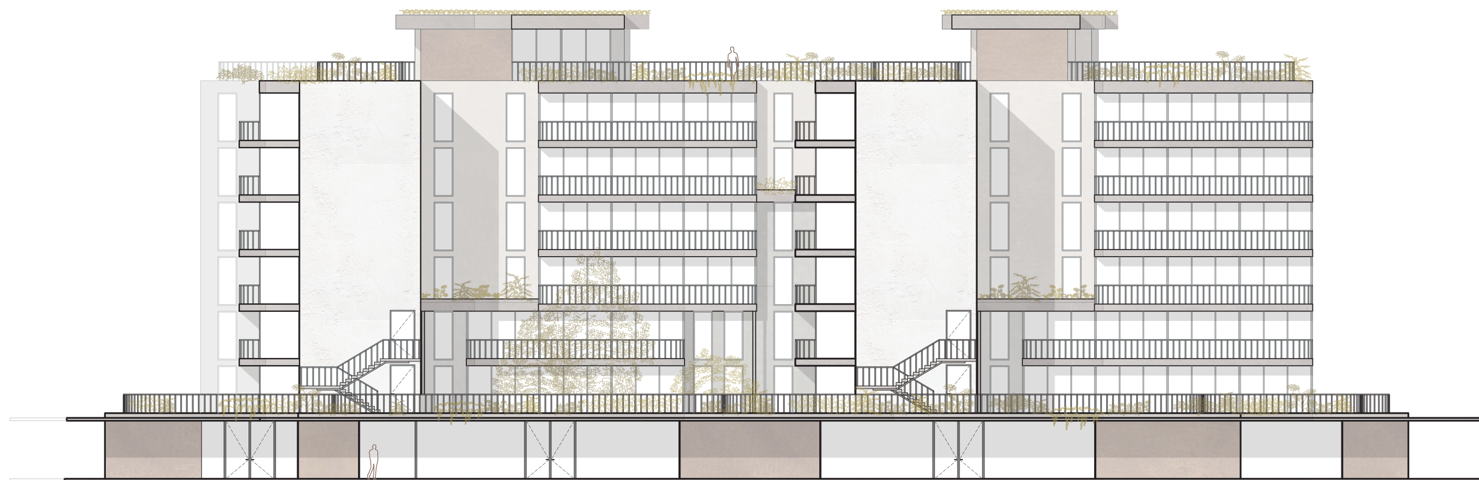
ALÇADO SUL
