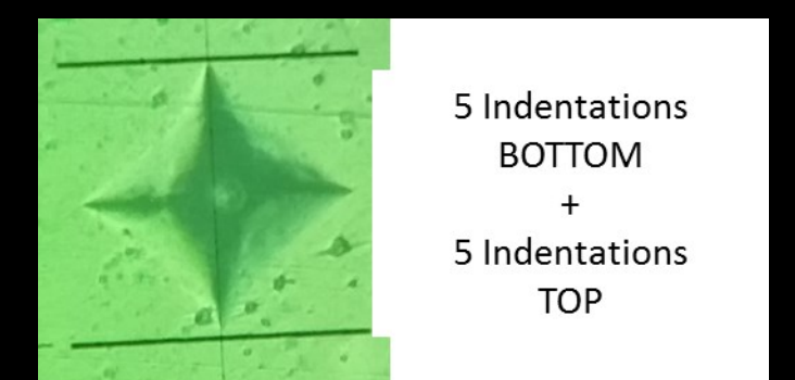
Fig. 5—Indentation
