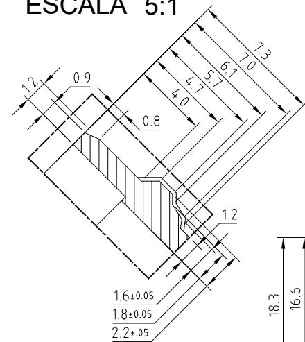
SECÇÃO DD ESCALA 5:1
