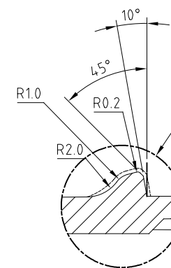
PORMENOR Y ESCALA 5:1
