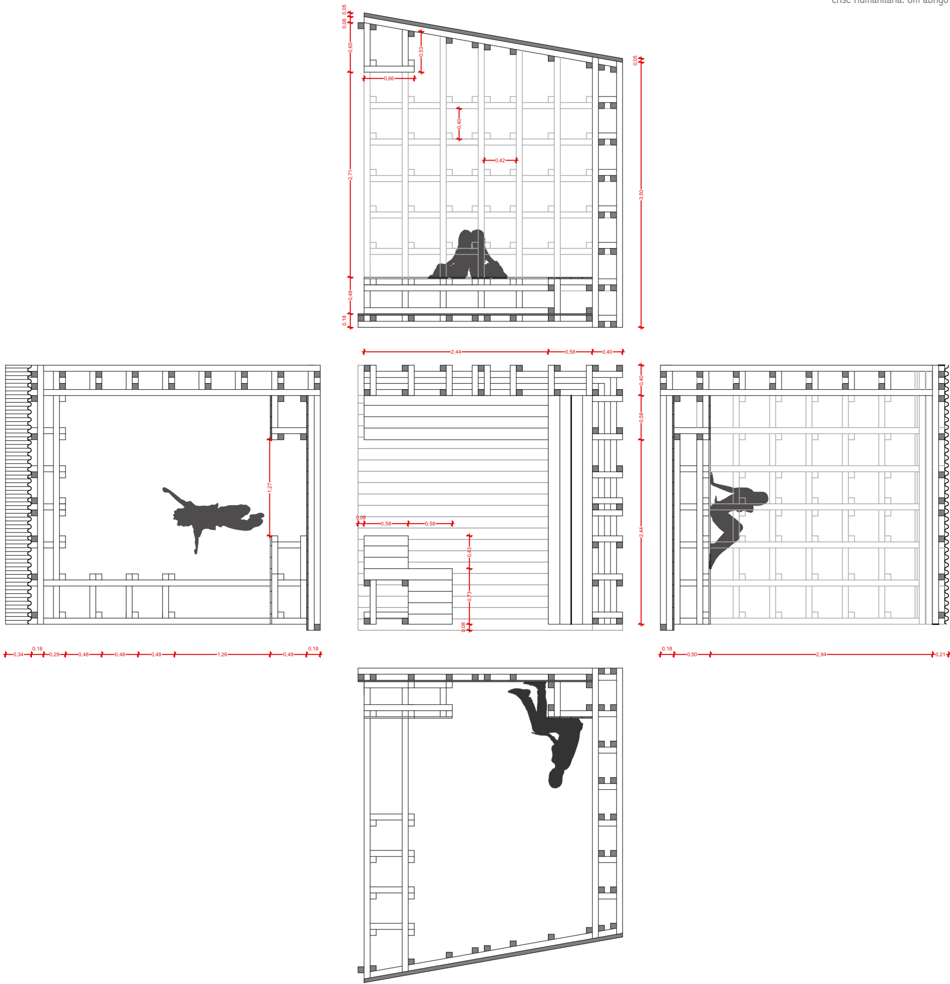
Módulo A-2: Desenho de pormenor e axonometria
