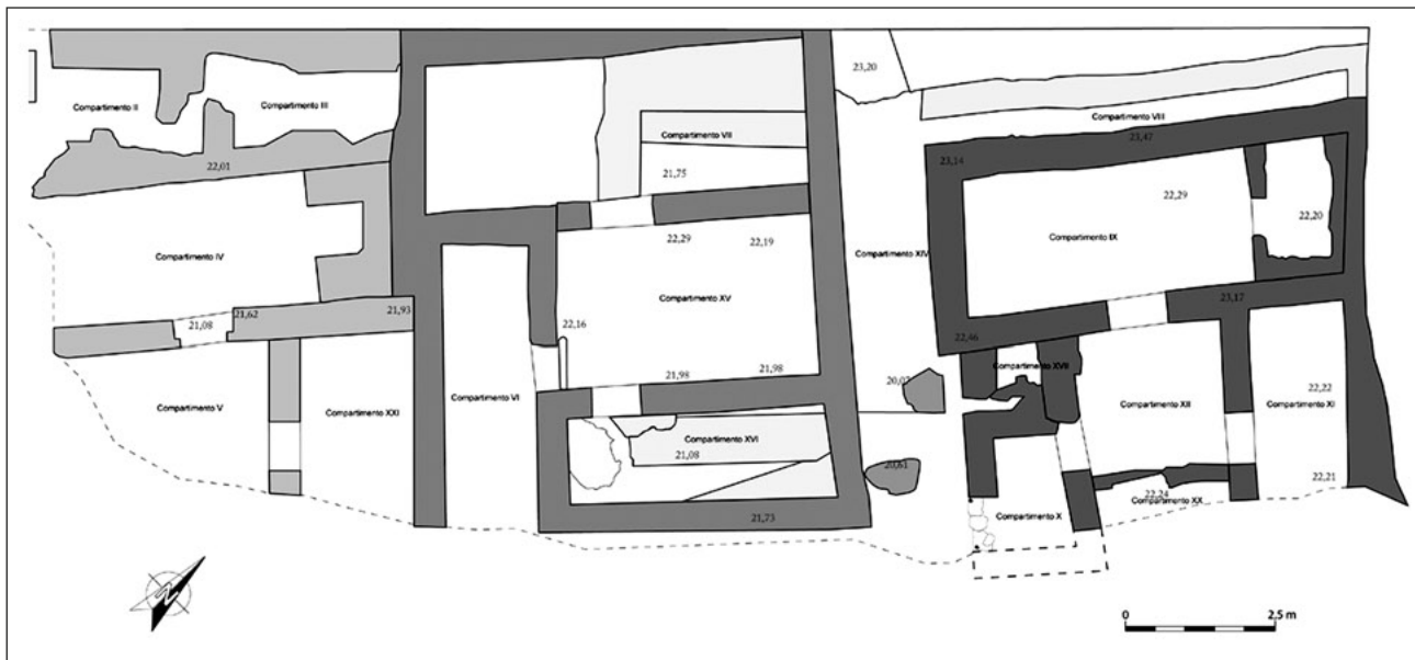
fig. 2 – Planta de las viviendas del siglo XII de la Hospedaria Beira Rio.
