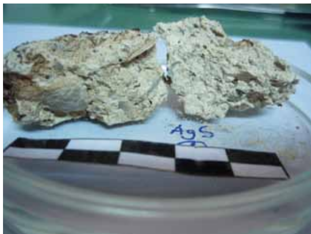
Exemplo do exame à lupa binocular. Amostra A: argamassa de cal branca com lamelibrânquios de grandes dimensões e muito abundantes. O inerte utilizado apresenta grande dispersão granulométrica, com predominância para os cristais de grande dimensão, sendo raros os minerais de cor escura.
