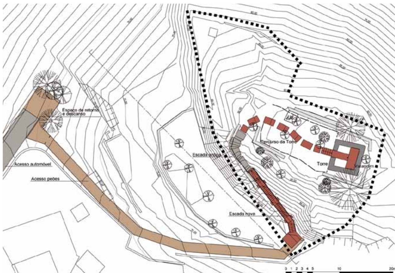
Planta geral da intervenção com delimitação da “área de grande sensibilidade arqueológica”.
