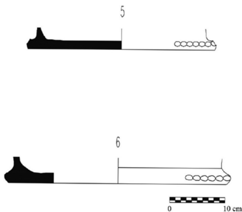
Formas cerâmicas. Fragmentos de fundos.
