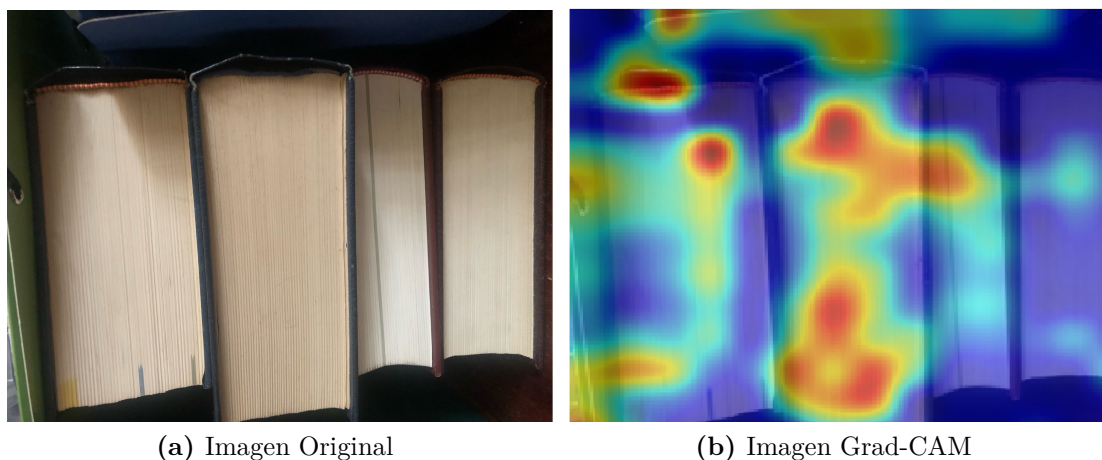
Figura 2.19: Aplicación Grad-CAM a la Clasificación de Libros Apilados. Fotografía suministrada por Ana Guerrero Tamayo.
