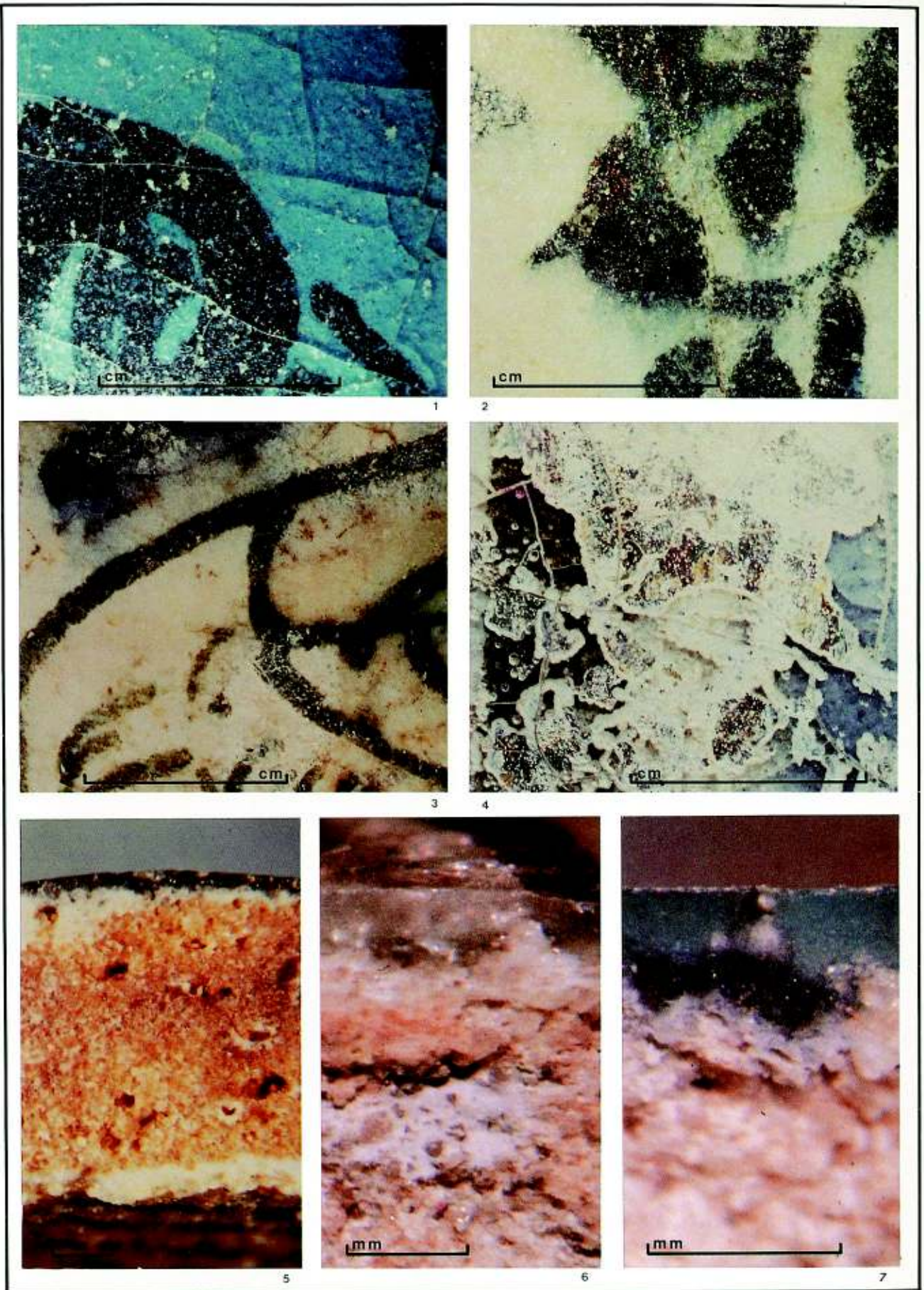
Fig. 7 - Aspect de surface : 1. céramique à décor noir sous glaçure bleu (Avignon, Petit Palais, n° 339); 2. céramique à décor bleu sous glaçure incolore (Carcassonne); 3. céramique à décor bleu et noir sous glaçure incolore (Avignon, Petit Palais, n° 887 et 1436); 4. céramique à décor bleu et noir sous glaçure incolore irisée (Avignon, Petit Palais, n° 651. non mouillée pour la photographie).
