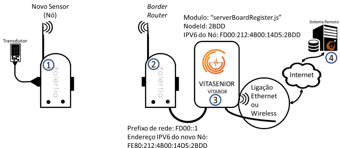
Figura 32 – Nó da rede e border router. Exemplo de associação do um novo nó
