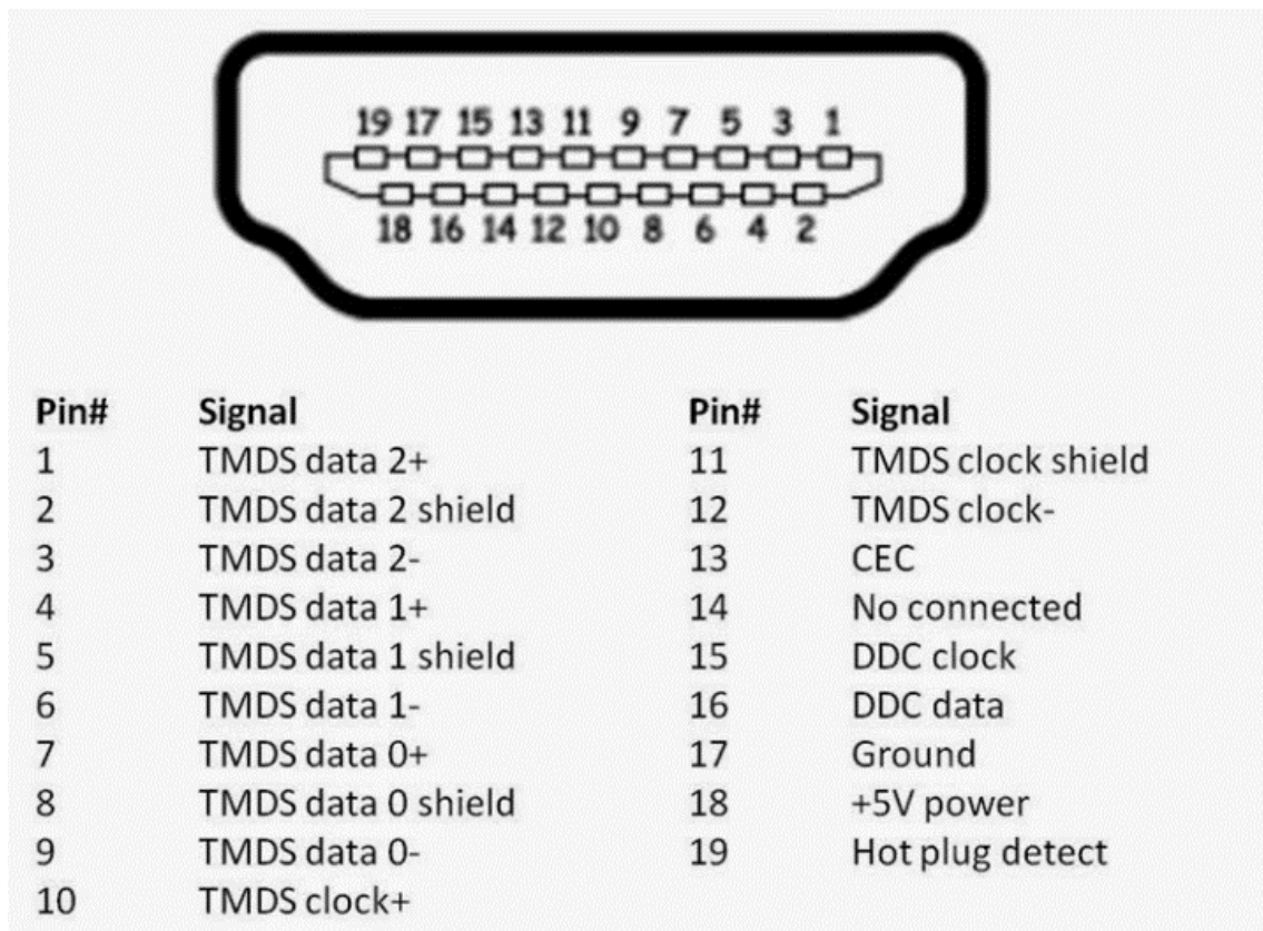
Figura 11 - Descrição dos pins da ligação HDMI 18
