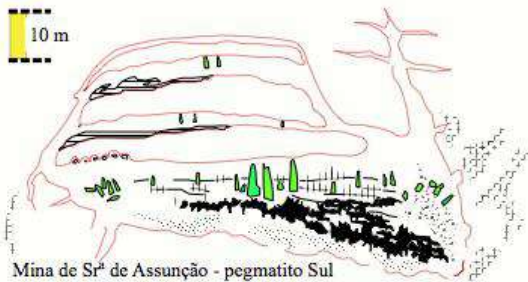
Mina de Sr a de Assunção - pegmatito Sul Corte N10°E exposto a E Encaixante: Granito porfiróide essencialmente biotítico
