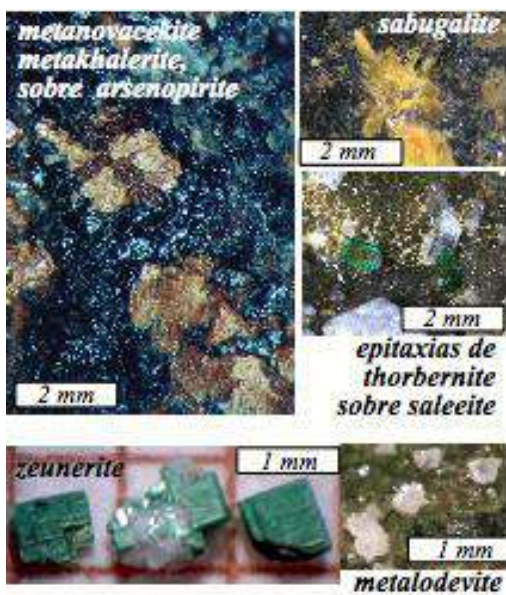
Figura 20 Diversidade de minerais indicadores de radiação anómala num pegmatito de Senhora de Assunção em Viséu – microfotografias de sais supergénicos.
