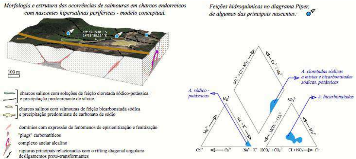
Figura 34 Generalização 3D do posicionamento de emergências sua feição hidroquímica e escorrências observadas em Salinas (Gabela); bloco diagrama visto de SW para NE.
