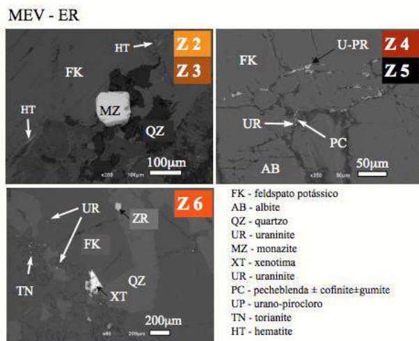
Figura 26 Mineralogia da matriz envolvente dos megacrístais de feldspato, nas zonas de enrubescimento diferenciado relacionadas com variações da saturação de cor rubra e com o risco e magnitude de exposição à radioatividade natural. Ocorrência da Pedreira de Casas de Monforte, Chaves, Trás-os-Montes.
