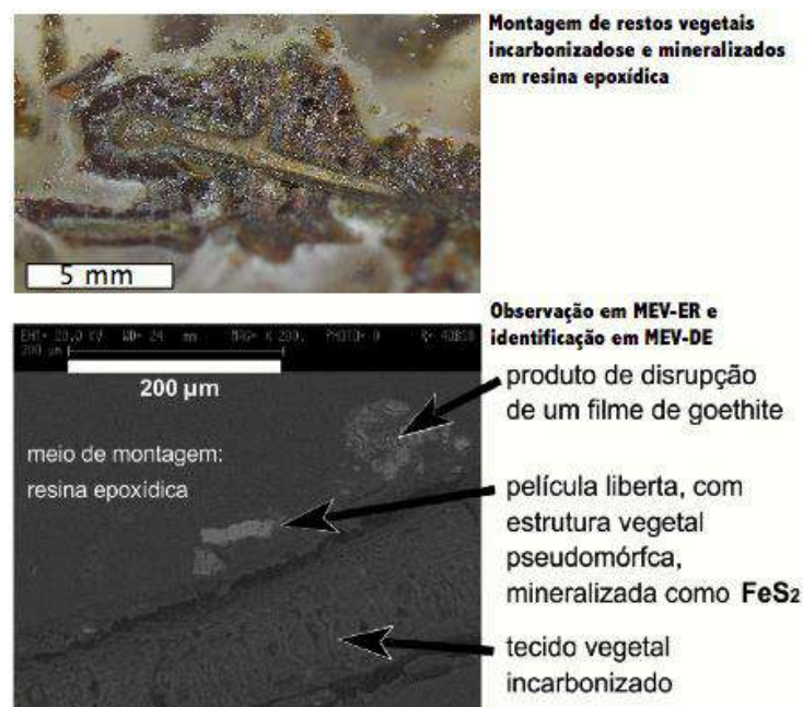
Figura 7 Produtos de evolução necrótica de tecidos vegetais: goethite de ruptura de placas, tecido orgânico em decomposição/incarbonização e piritização de restos vegetal (microambiente redutor desencadeado pela diminuição de O_2 consumido na evolução da matéria orgânica). Observações em MEV-ER e MEV-DE.
