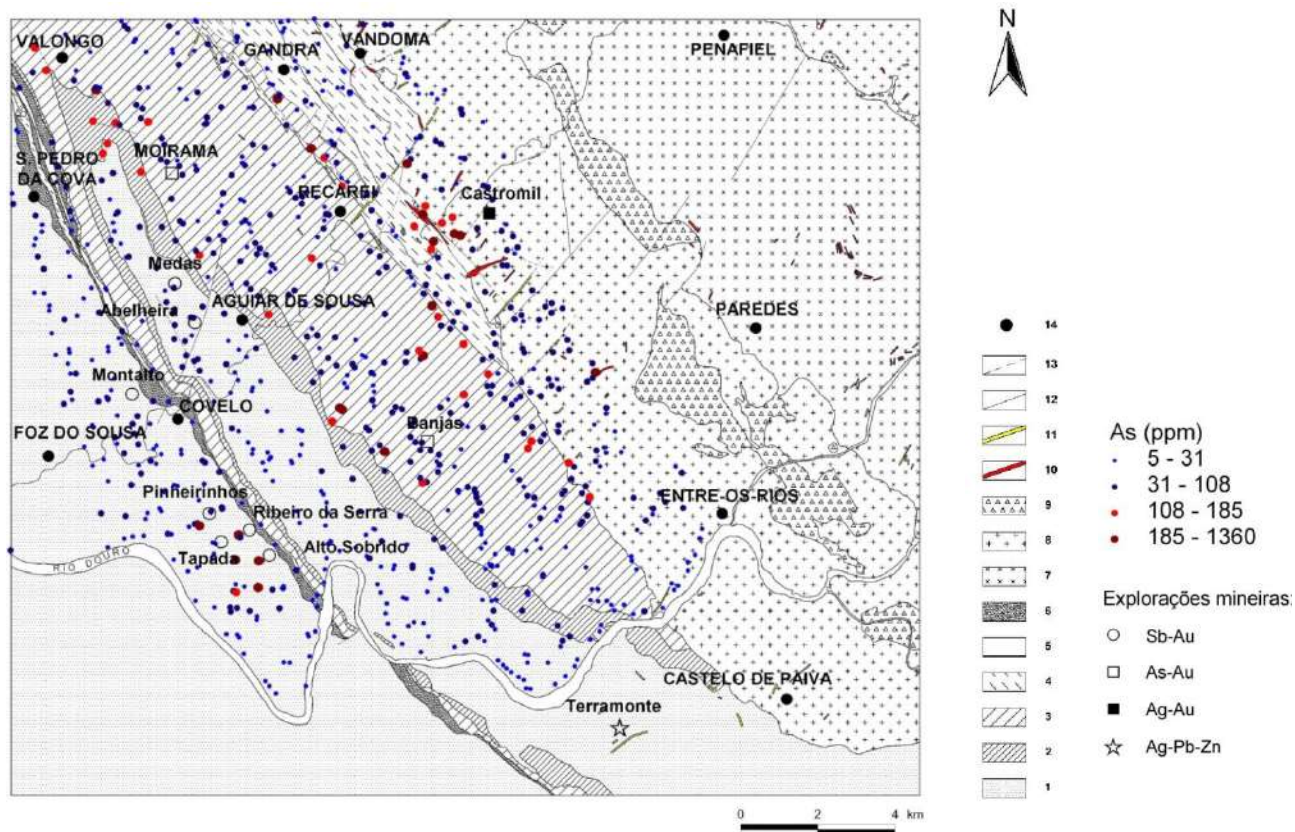
Figura 7 Distribuição da concentração de As nos de sedimentos de corrente de Valongo. 1-Complexo Xisto- Metagrauvaquico- Câmbrico; 2- quartzitos e xistos argilosos intercalados- Arenigiano; 3- Xistos ardosíferos- Lanvirniano a Landeiliano; 4- Intercalações de xistos, grauvaques e quartzitos- Silúrico; 5- Quartzitos, e xistos argilíticos- Devónico, 6- Conglomerados e quartzitos- Carbónico, 7- Granito médio a grosseiro, porfiróide biotítico>moscovítico; 8- granodiorito de grão médio, porfiróide, moscovítico biotítico, 9- granodiorito de grão fino, porfiróide, biotítico>moscovítico; 10- Filões de pegmatito, aplito e aplito-pegmatito; 11- Filões de quartzo; 12-Falhas e cavalgamentos; 13- Falhas prováveis; 14- Localidades.
