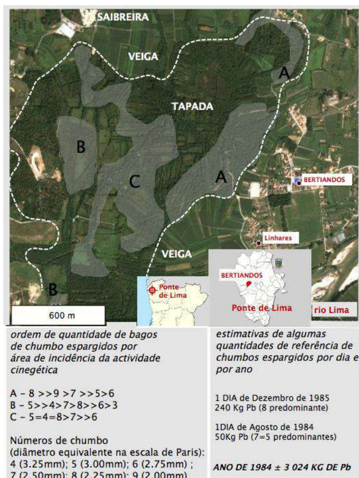
Figura 14 Perímetro das Lagoas de Bertiaundos e S. Pedro de Arcos com indicadores da aspersion de granalhas de chumbo de origem cinegética.
