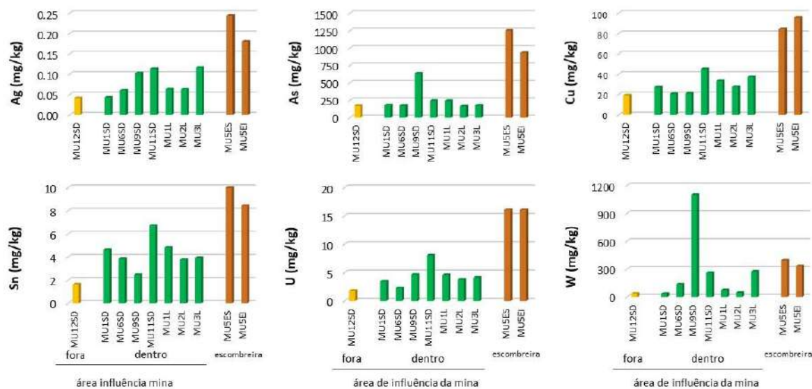
Figura 4. Diagramas de variação para os sedimentos de corrente e escombreiras da área mineira de Murçós.
