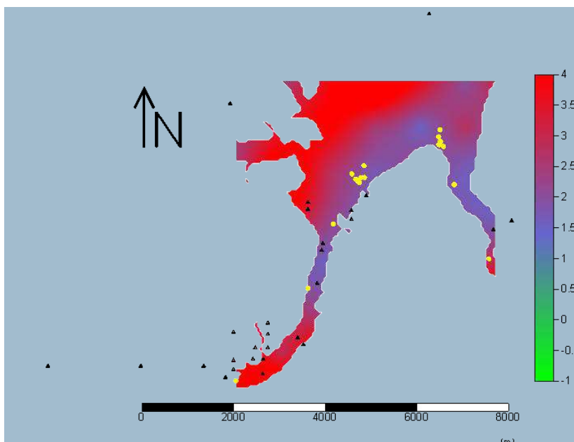
Figura 7. Mapa estimado por Krigagem com deriva externa (KED).
