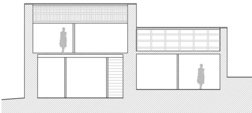
Sección AB
