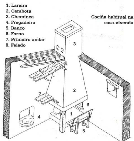
Fig.70. Lareira típica galega.
