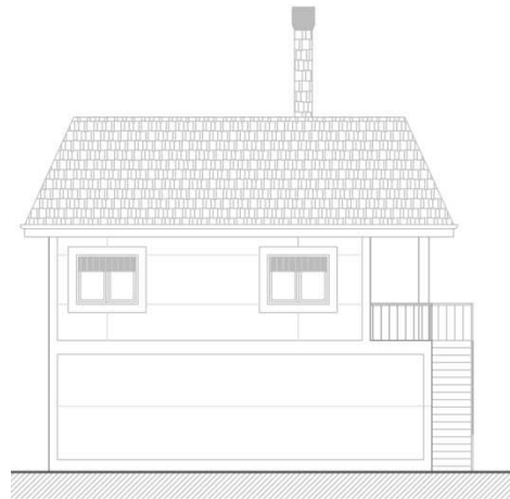
Alzado Oeste
