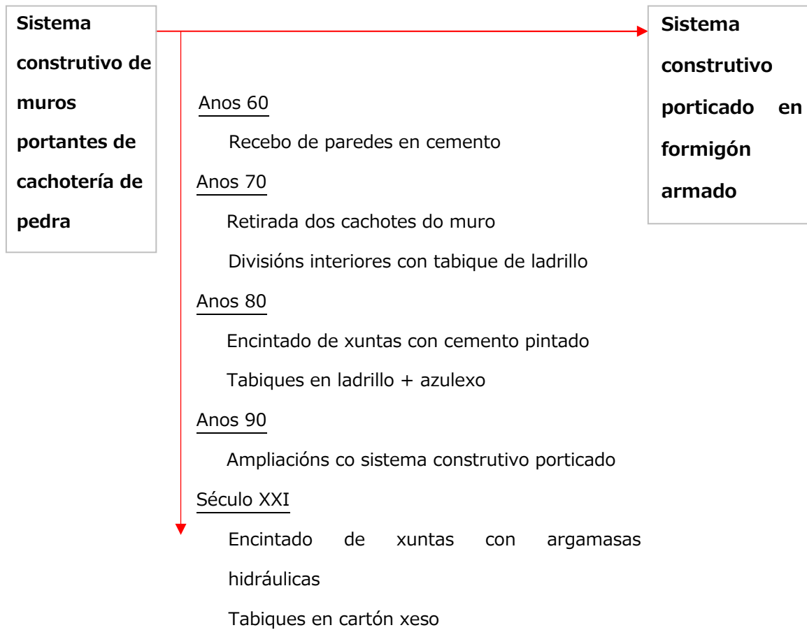
Fig. 165. Esquema resumen da transformacións dos elementos verticais
