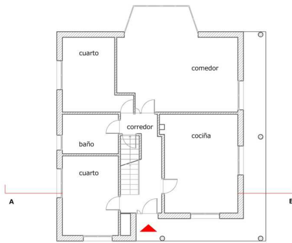
Planta alta
