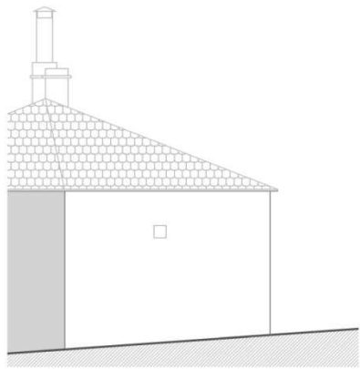
Alzado Este
