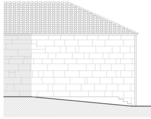
Alzado oeste
