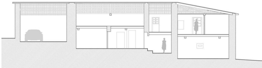
Sección AB
