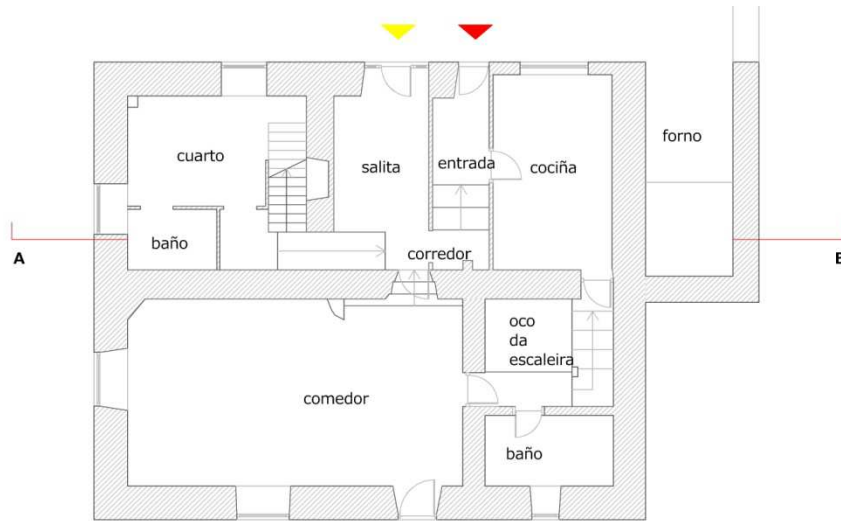
Planta baixa
