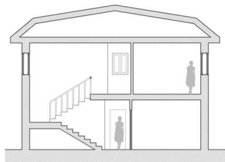
Sección AB
