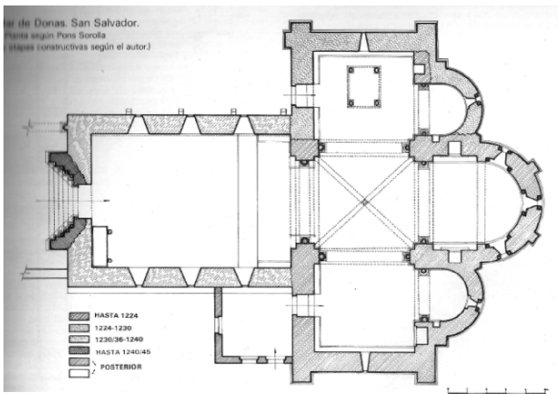
Fig.3. Planta da Igrexa de Vilar de Donas segundo as etapas constructivas.
