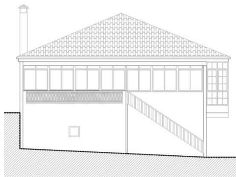
Alzado Sur
