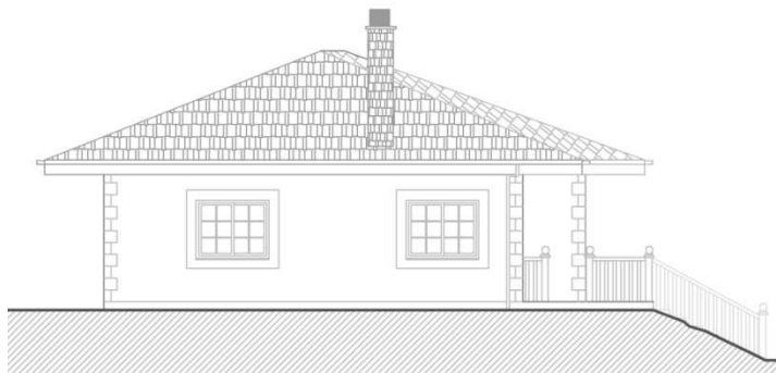
Alzado Sur
