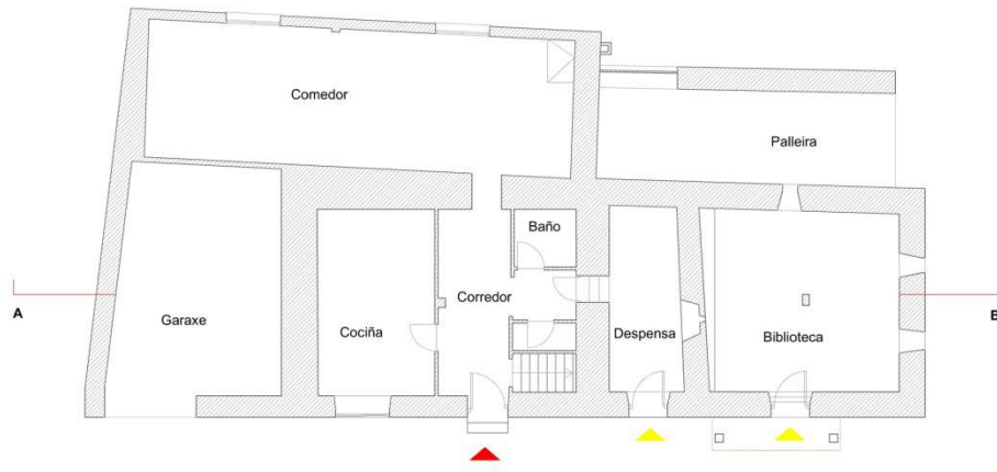
Planta Baixa
