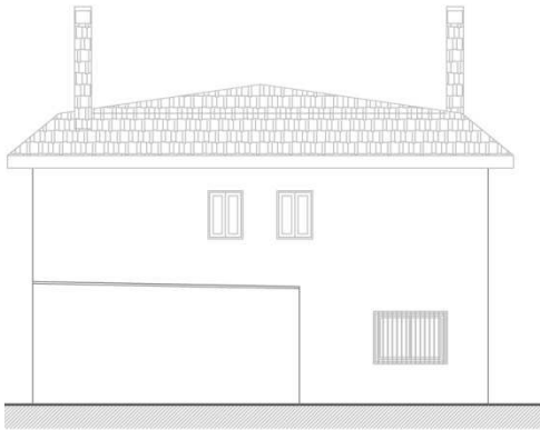
Alzado Norte
