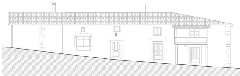
Alzado Este
