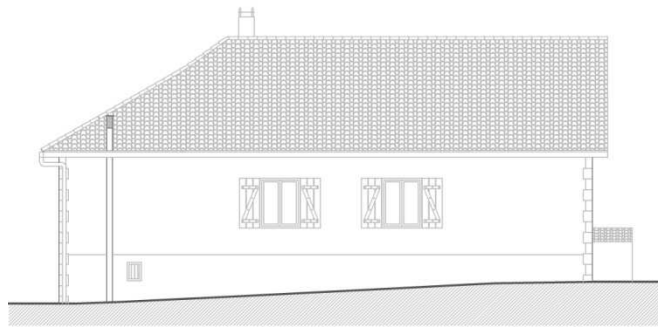
Alzado Norte
