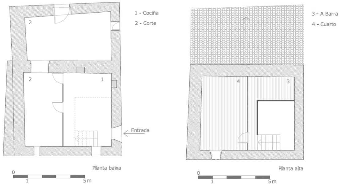
Fig.68. Planta baixa e alta da casa de Arcovello no século XX. (reconstrucción)
