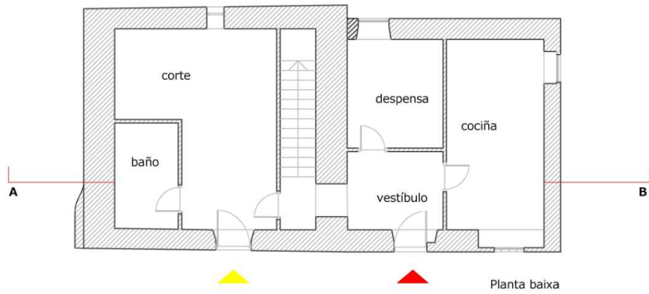
Planta baixa
