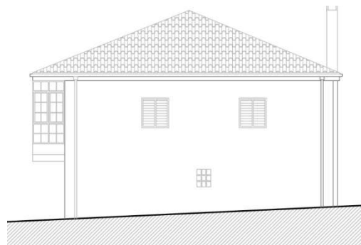
Alzado Norte
