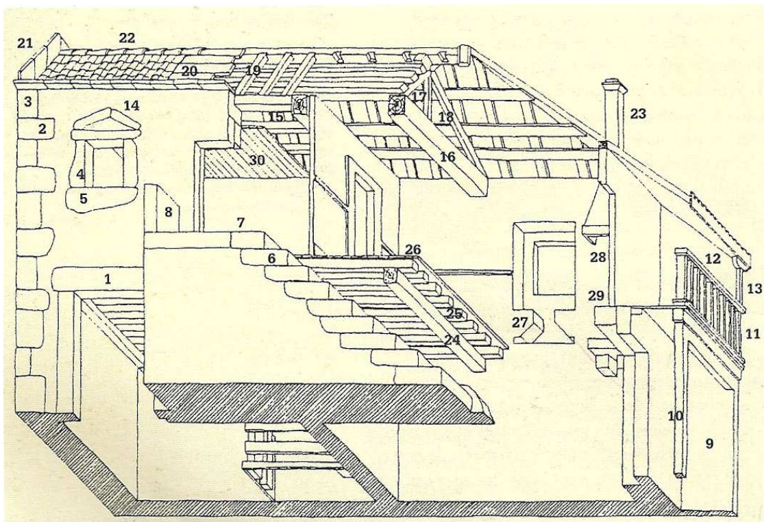
Fig.62. Casa-vivenda tradicional Fonte: (Caamaño, 2006.a, p.104)
