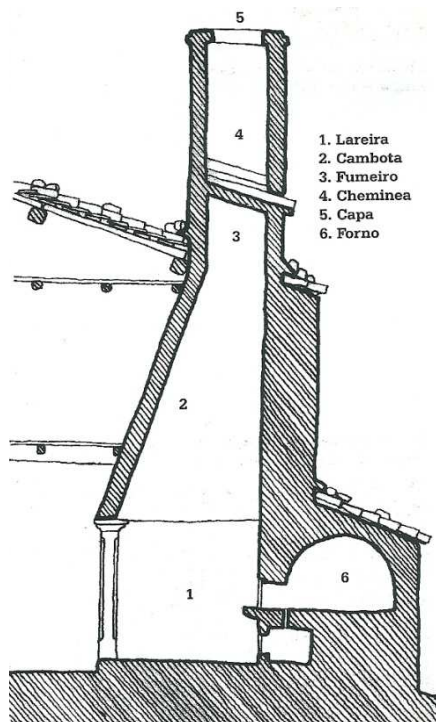
Fig.71. Lareira típica galega
