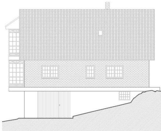
Alzado Este
