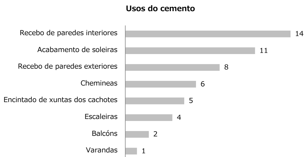
Fig.150. Táboa uso do cemento nos elementos construtivos das casas de Vilar de Donas
