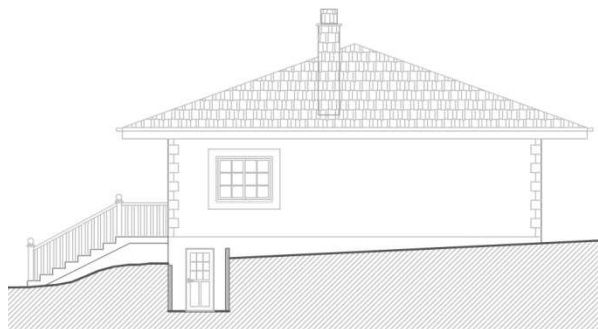
Alzado Norte
