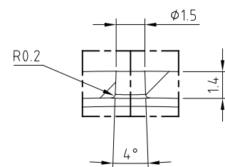
PORMENOR X ESCALA 5:1
