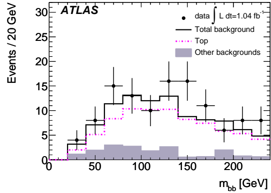
(d) m_{\ell\ell} sidebands, E_T^{\text{miss}} < 50 GeV, tagged sample.
