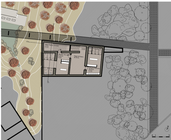
Planta do Piso -1.
