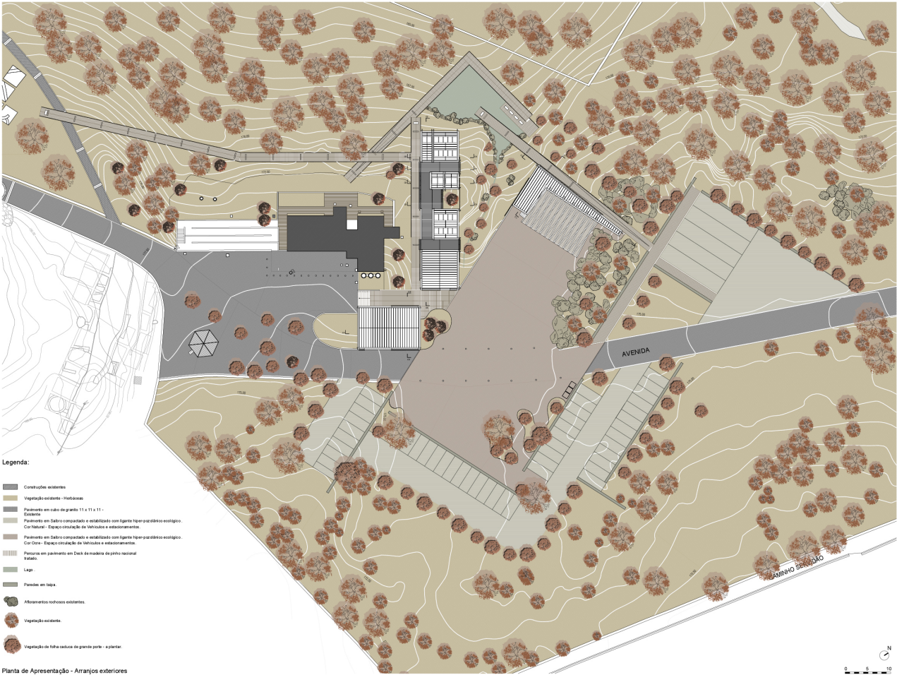
Planta de Apresentação - Arranjos exteriores
