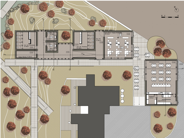
Planta do Piso 0.
