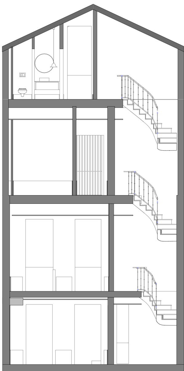
Imagem 156| Corte Transversal Escada de Serviço
