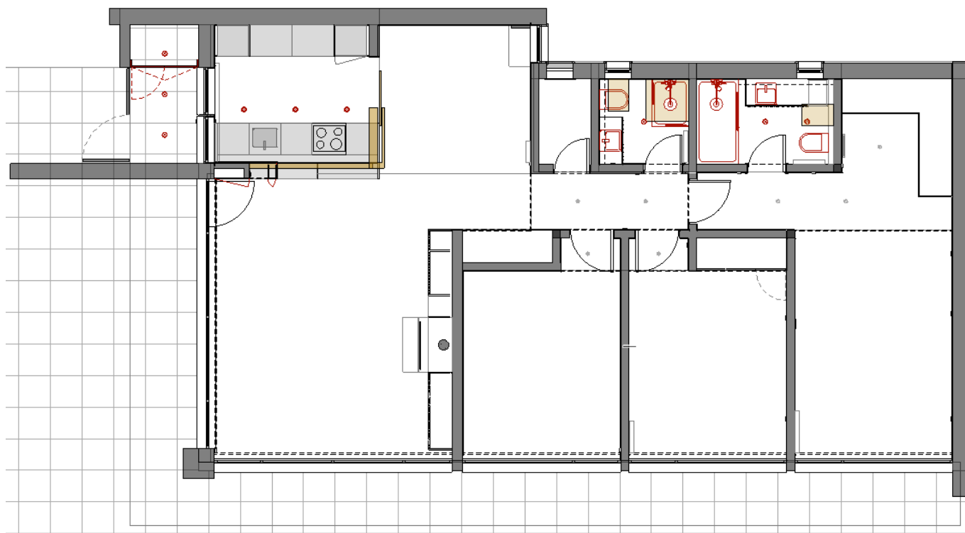
Imagem 40 | Planta V/A Casa de Férias em Moledo
