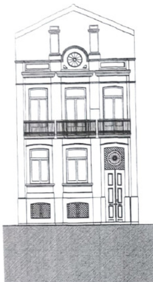
Imagem 114 | Alçado Frontal Pré-existência Villa Coworking
