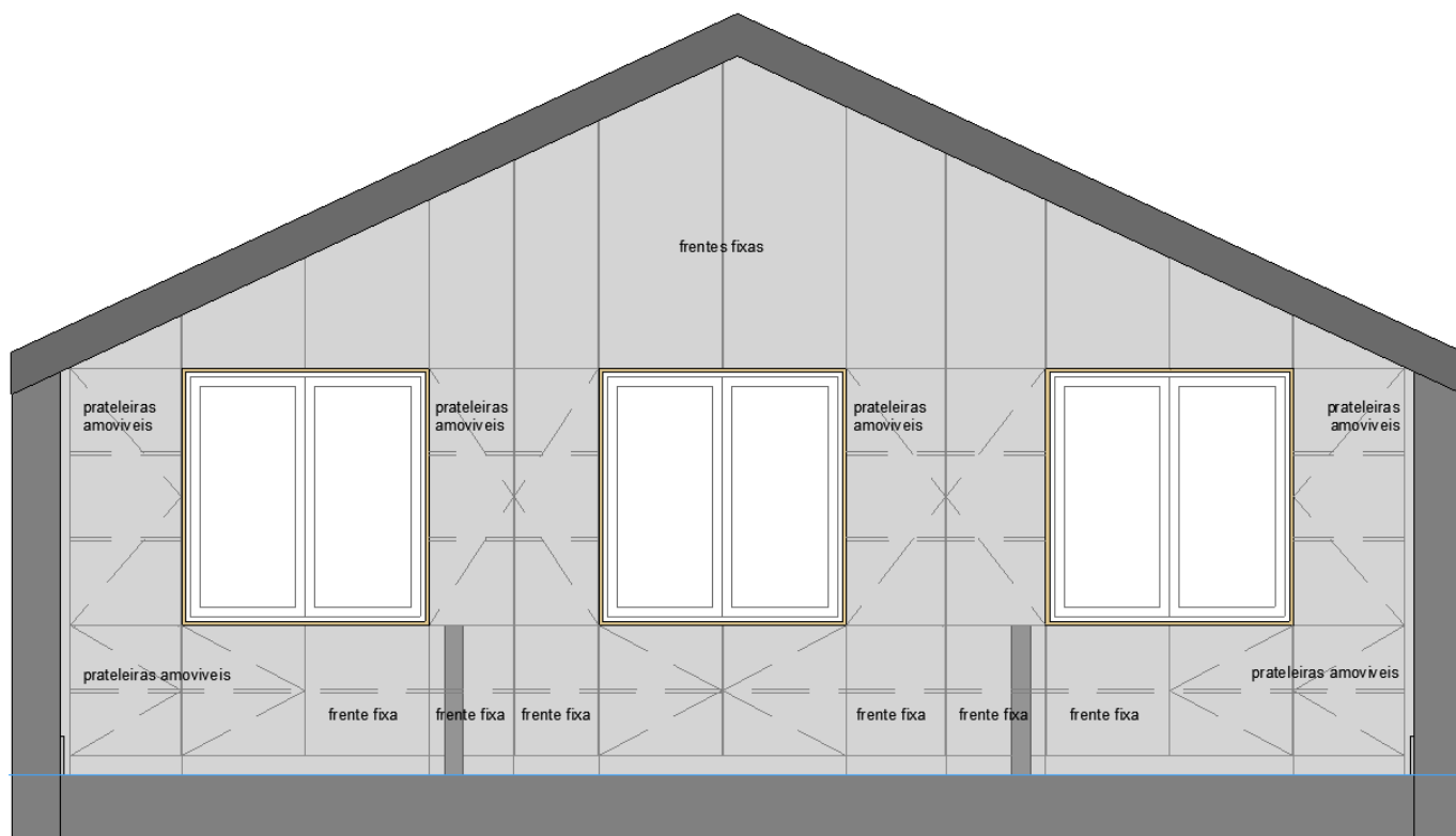
Imagem 150 | Alçado Frontal Móvel Fixo de Arrumos
