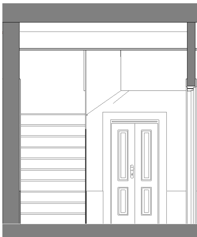
Imagem 142 | Alçado Frontal Escada de Ligação Piso 0 a Piso 1
