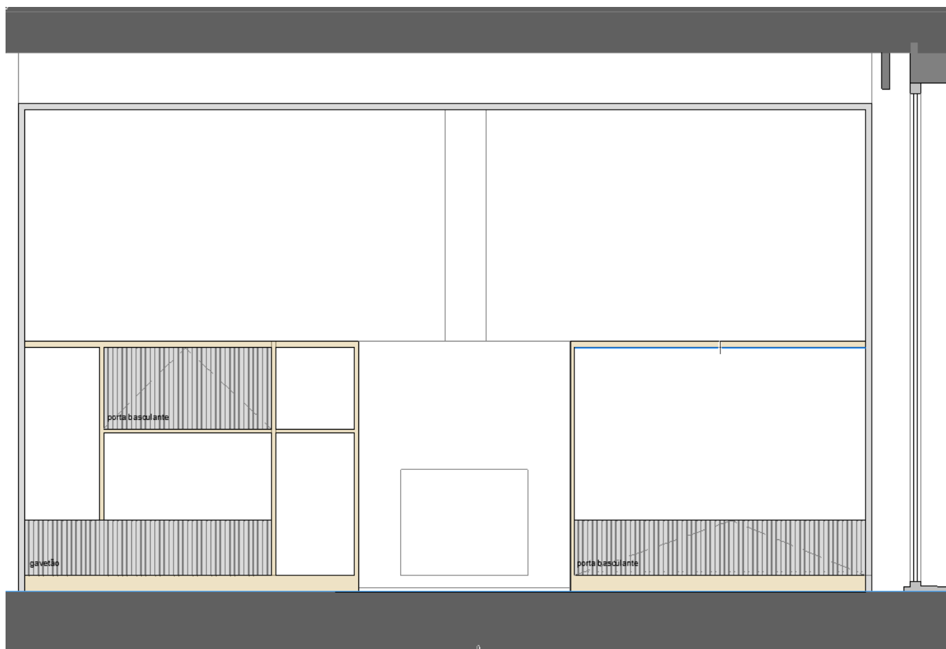
Imagem 53 | Alçado Frontal Estante Sala
