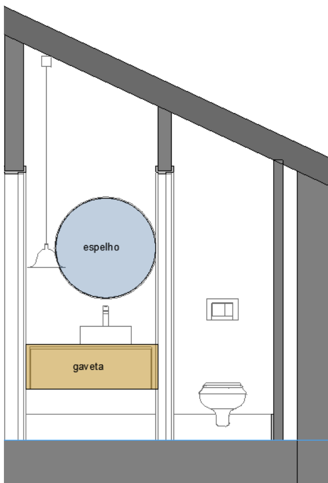
Imagem 154| Alçado Frontal Móvel WC
