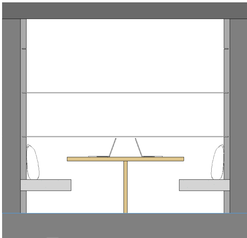
Imagem 153| Corte Transversal Phone Booths
