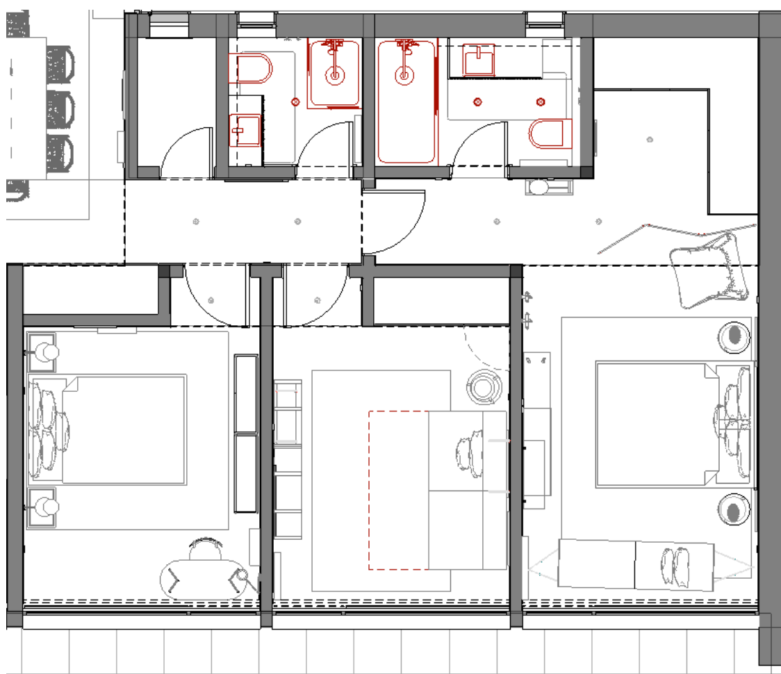
Imagem 75 | Pormenor Planta Zonas Privadas Casa de Férias em Moledo
