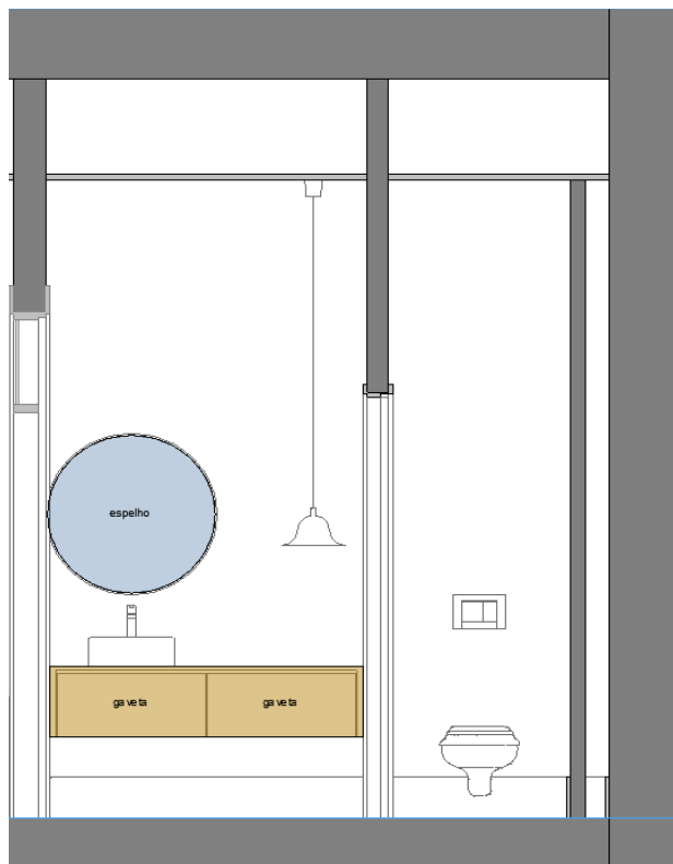
Imagem 141 | Alçado Frontal Móvel WC
