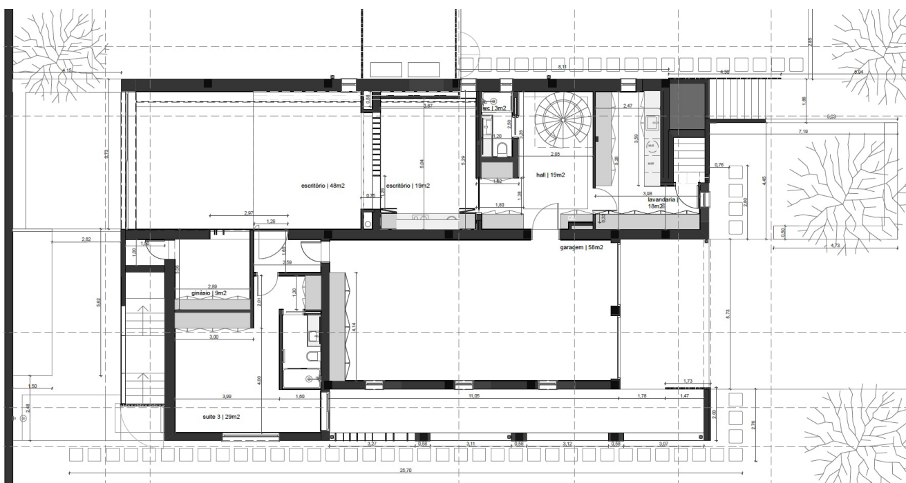
Imagem 06 | Planta piso 0 Casa na Praia
