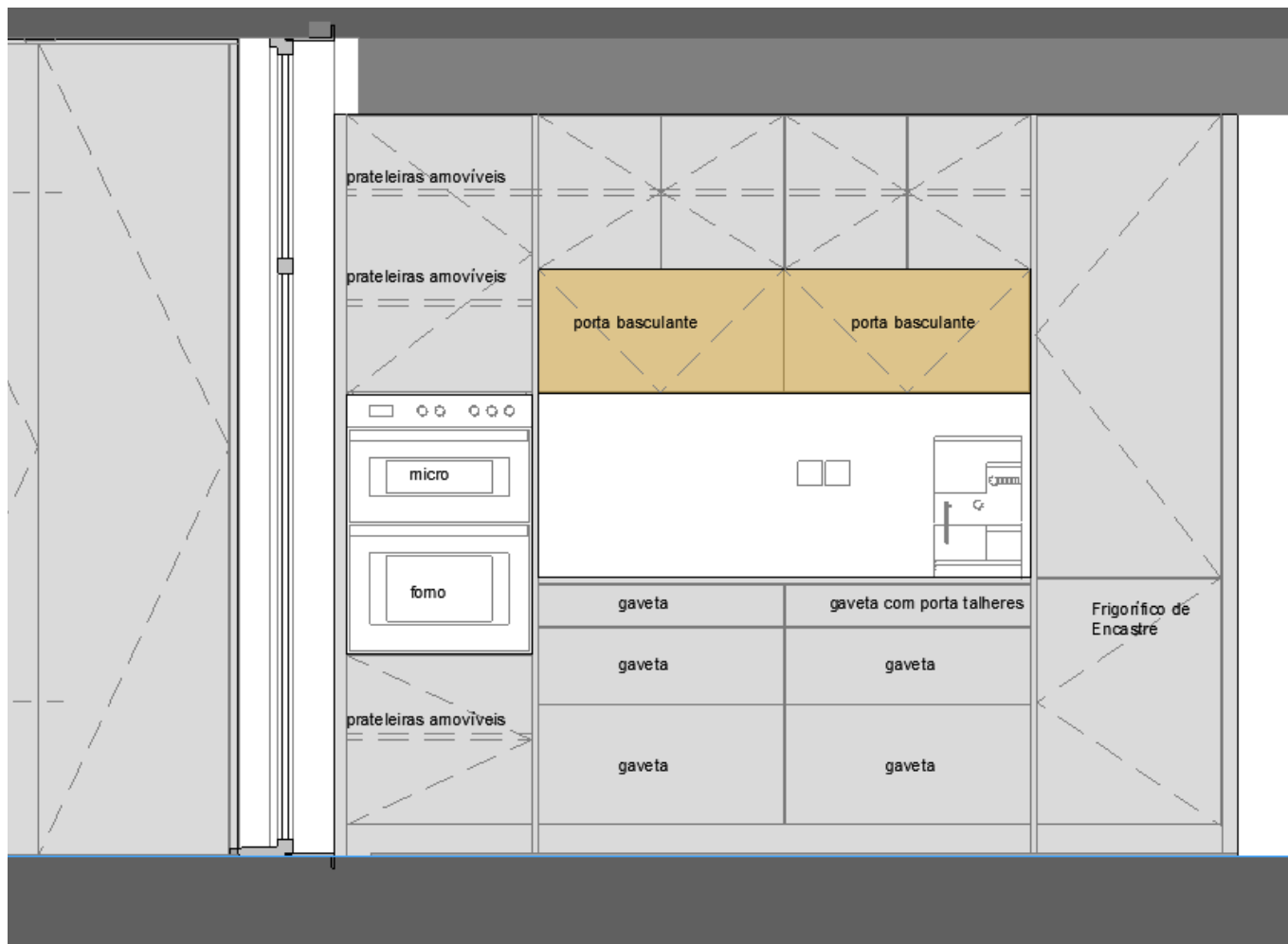
Imagem 45 | Alçado Frontal Módulos Altos Cozinha
