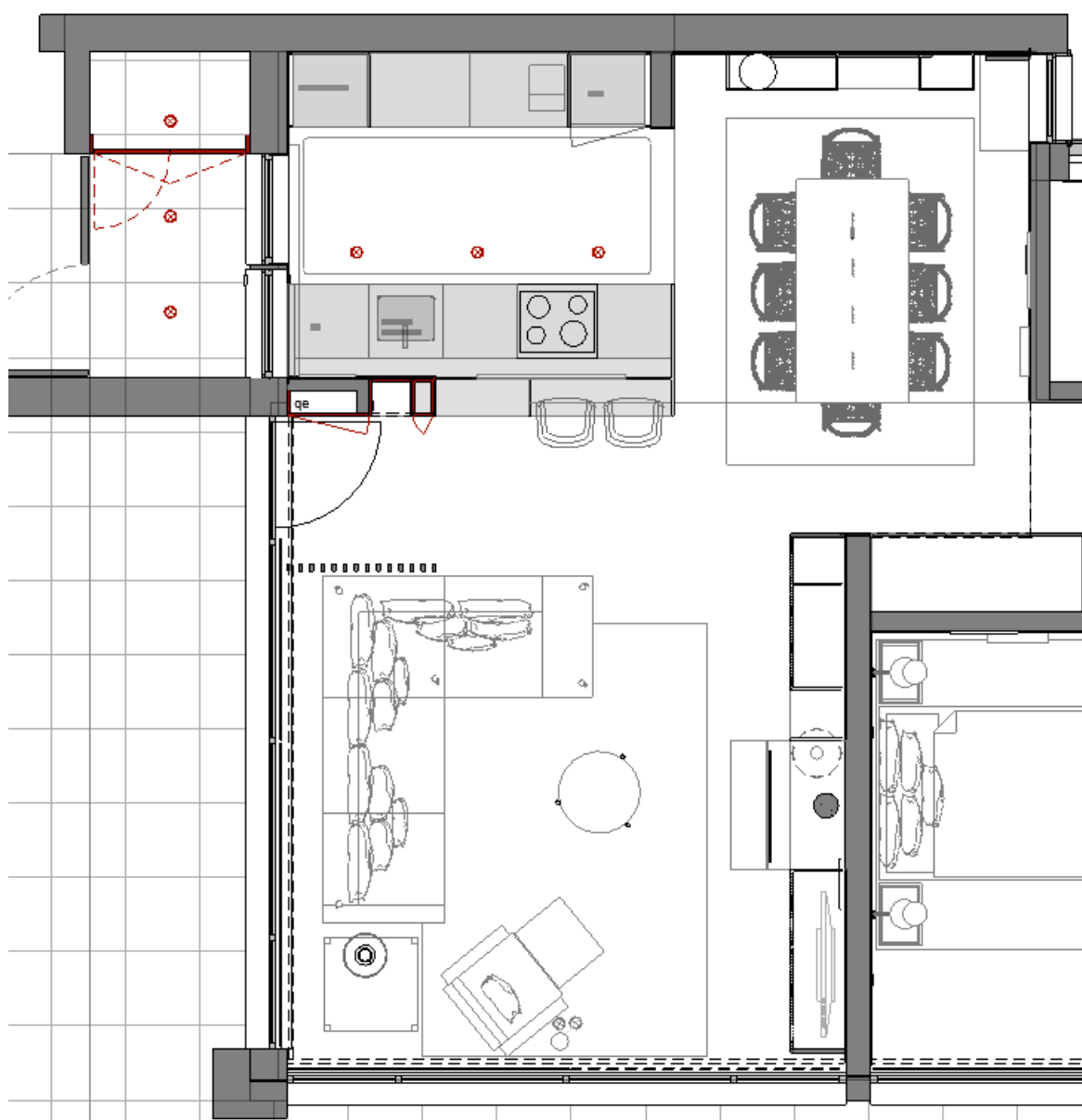
Imagem 44 | Pormenor Planta Zonas Comuns Casa de Férias em Moledo
