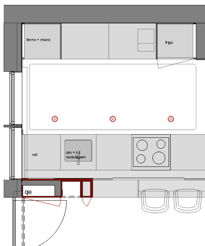
Imagem 51 | Planta Cozinha
