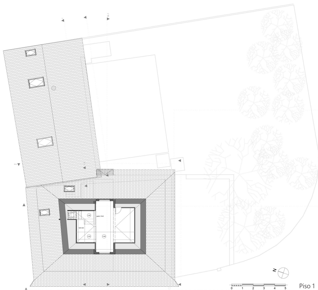
Imagem 22 | Planta Piso 1 Casa do Eirado
