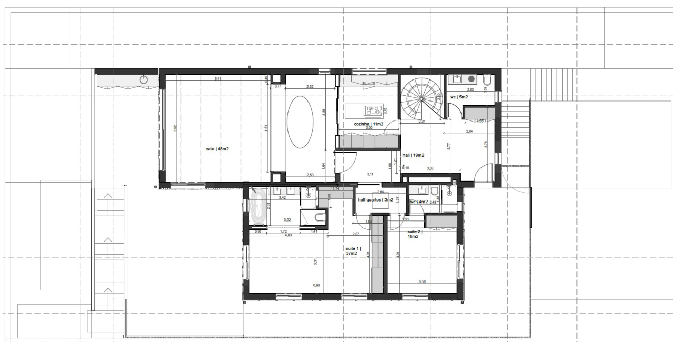
Imagem 07 | Planta piso 1 Casa na Praia
