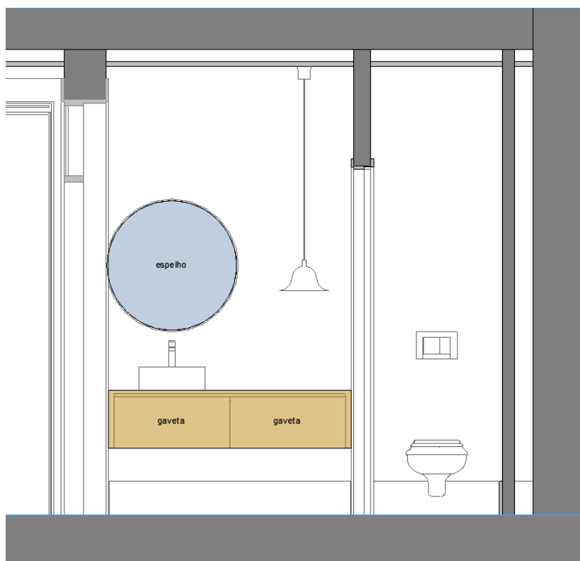
Imagem 135 | Alçado Frontal Móvel WC
