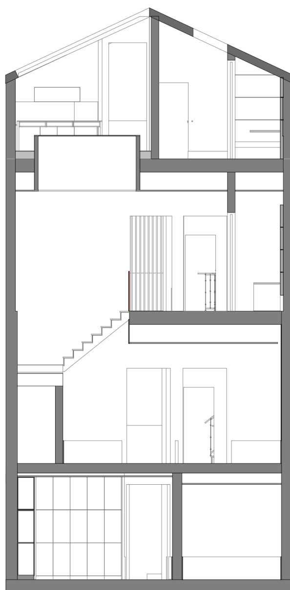
Imagem 157| Corte Transversal Claraboia Central
