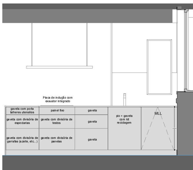
Imagem 46 | Alçado Frontal Bancada Cozinha
