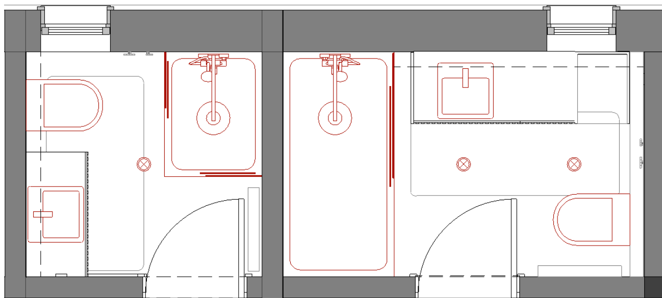
Imagem 104 | Planta WCs
