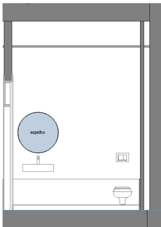
Imagem 147 | Corte Transversal WC
