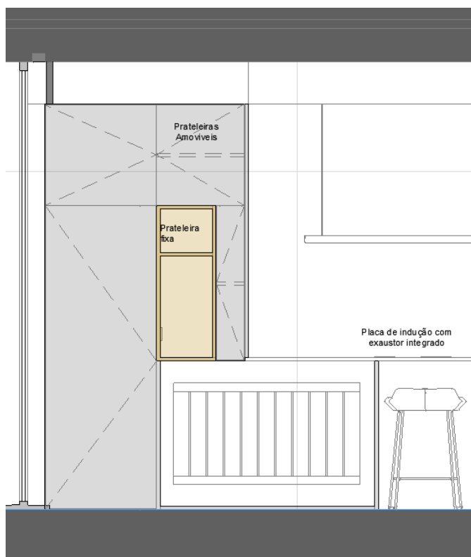
Imagem 54 | Alçado Frontal Móvel de Entrada
