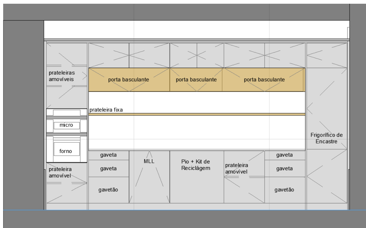
Imagem 137 | Alçado Frontal Módulos Altos Cozinha
