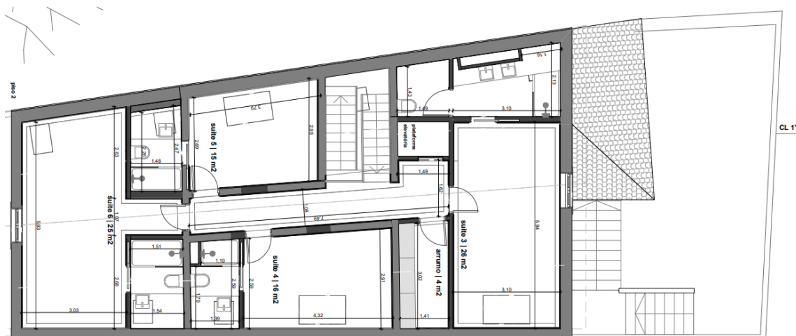
Imagem 15 | Planta Piso 2 Harbour Inn
