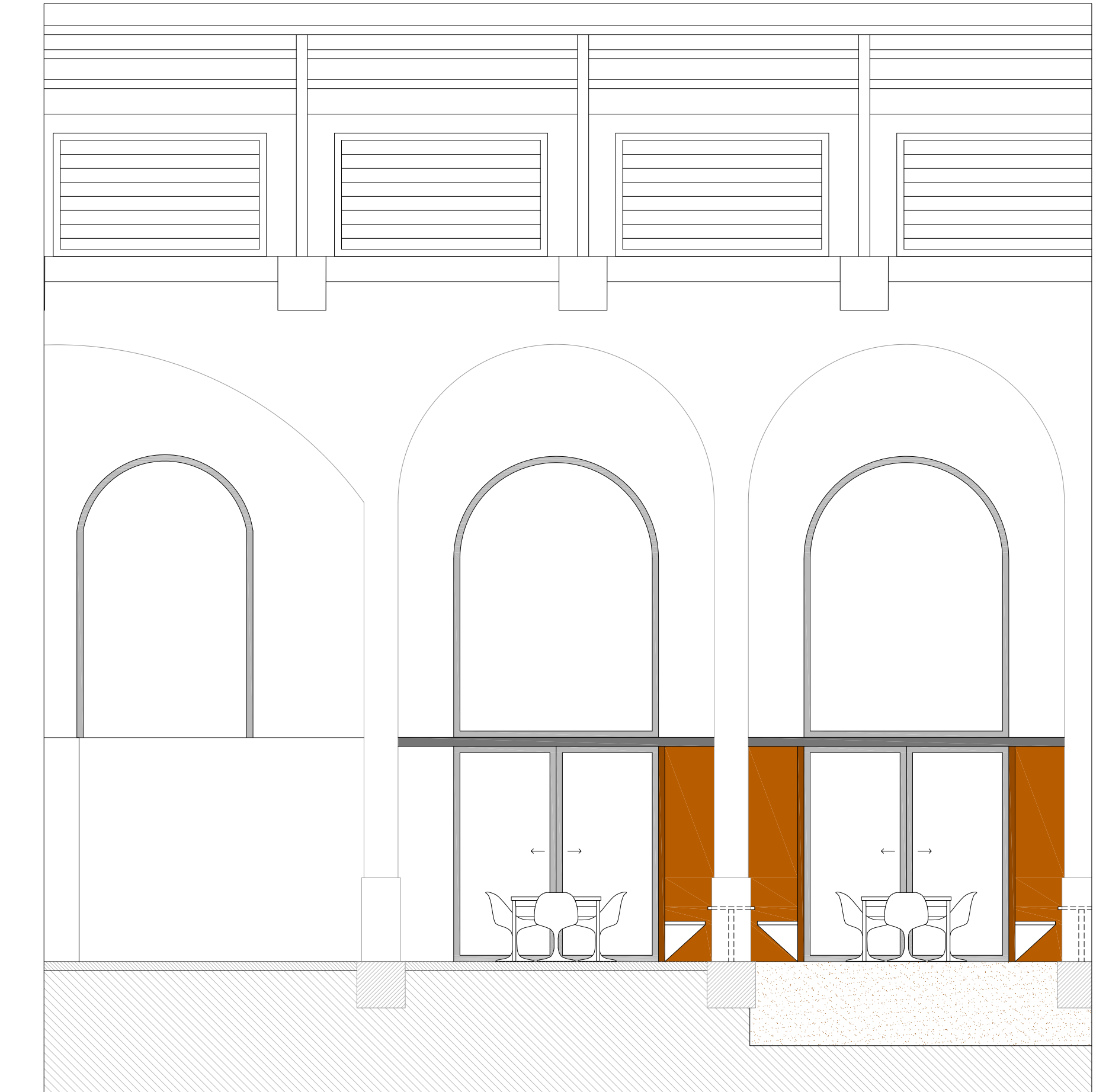
Corte BB
