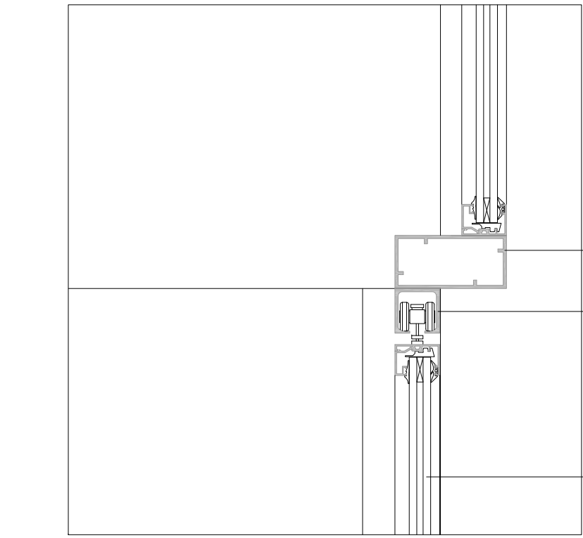
Detalhe_P1E_Esc 1/5
