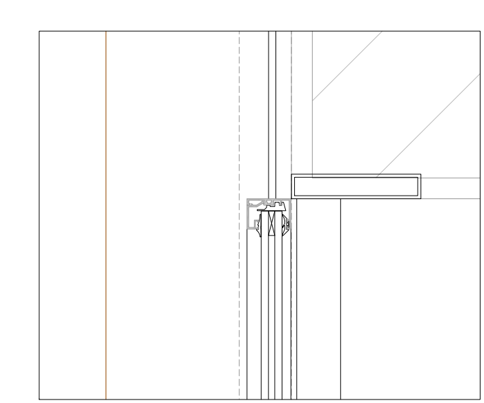
Detalhe_P1A_Esc 1/5
