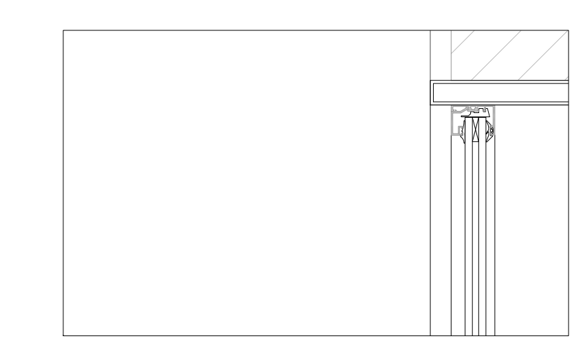
Detalhe_P1D_Esc 1/5
