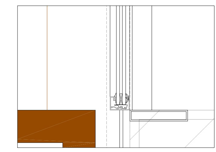
Detalhe_P1C_Esc 1/5
