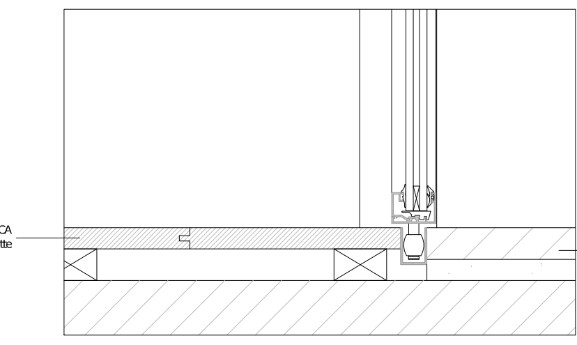
Detalhe_P1F_Esc 1/5
