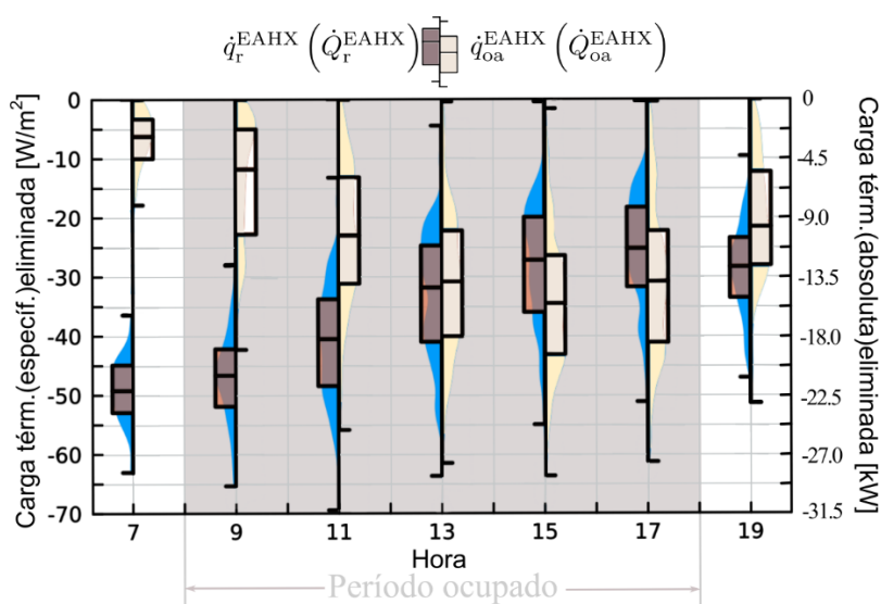
Figura 4. Gráficos de violín y de caja por hora para la eliminación de carga específica (y absoluta) en las oficinas— \dot{q}_r^{EAHX} ( \dot{Q}_r^{EAHX} )—y para la eliminación de carga específica (y absoluta) del aire exterior— \dot{q}_{oa}^{EAHX} ( \dot{Q}_{oa}^{EAHX} ). Obtenidos a partir de datos monitoreados (entre el 1 de junio y el 30 de septiembre; solo en modo de enfriamiento, T_{aL} < T_{a0} ; tasa de flujo nominal de 8000 m 3 /h; 450 m 2 de área de piso enfriado). El sombreado gris resalta el período de ocupación de las oficinas. Los ejes izquierdo y derecho representan la eliminación de carga específica y absoluta, respectivamente.
