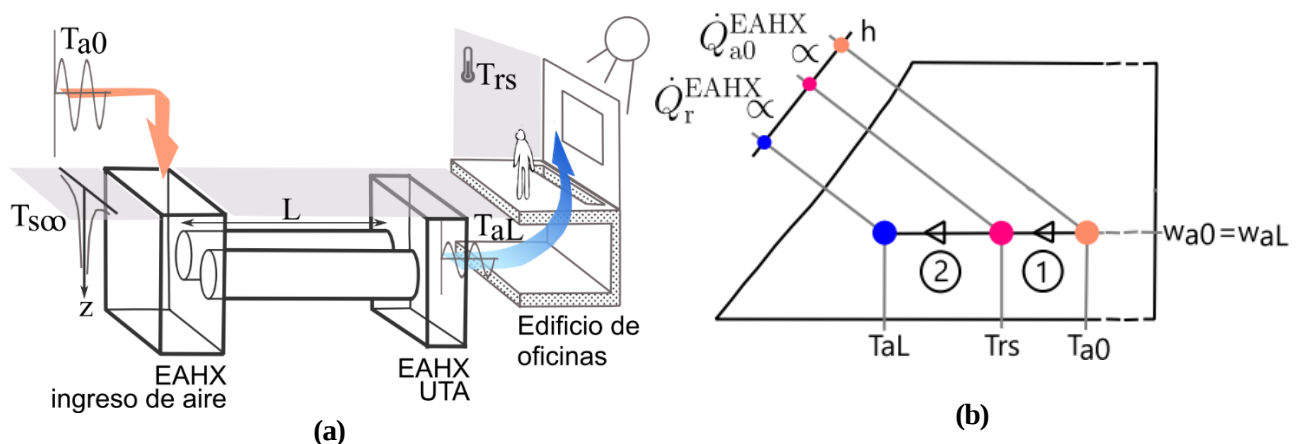
Figura 1. (a) Esquema de un EAHX para enfriamiento de un edificio de oficinas. (b) Detalle de un diagrama psicrométrico que esboza los procesos termohigrométricos con el aire desde el momento en que entra hasta que sale del EAHX. Las cargas ( \dot{Q} ) eliminadas del aire, proporcionales ( \propto ) a las diferencias de entalpía ( h ), están representadas para los subprocesos ① y ②.
