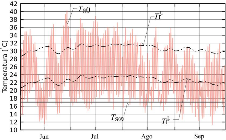
Figura 2. Series temporales de la temperatura del aire exterior ( T_{a0} , datos monitoreados); temperaturas de consigna superior e inferior de las oficinas ( T_r^U y T_r^L determinadas a partir de las Ecuaciones 3 utilizando datos de monitoreo); estimación de la temperatura del suelo no perturbado ( T_{s\infty} , determinada a partir de datos de temperatura media anual del aire exterior).
