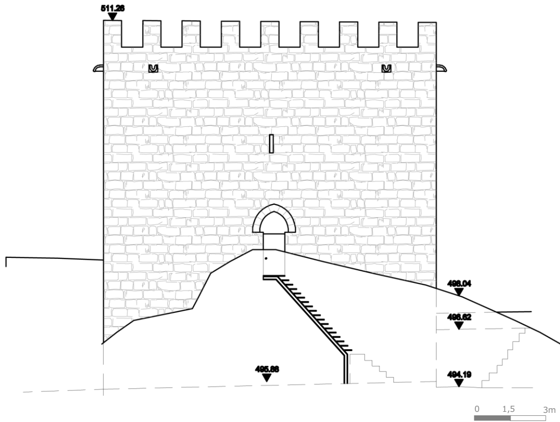
Alçado frontal.
