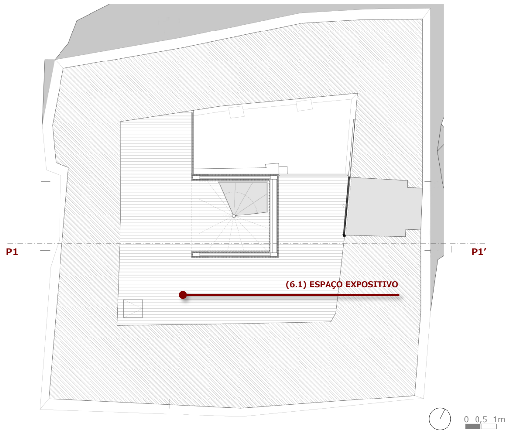
Figura 7.48. Planta do Piso 1. Adaptado pela autora.
