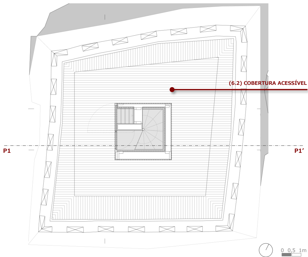
Figura 7.49. Planta do Piso 2. Adaptado pela autora.
