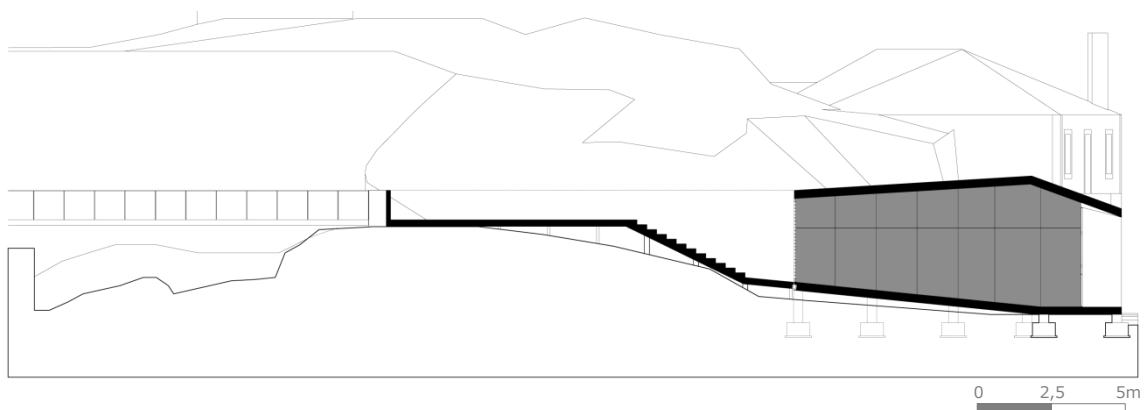
Figura 7.112. Perfil 1. Adaptado pela autora.
