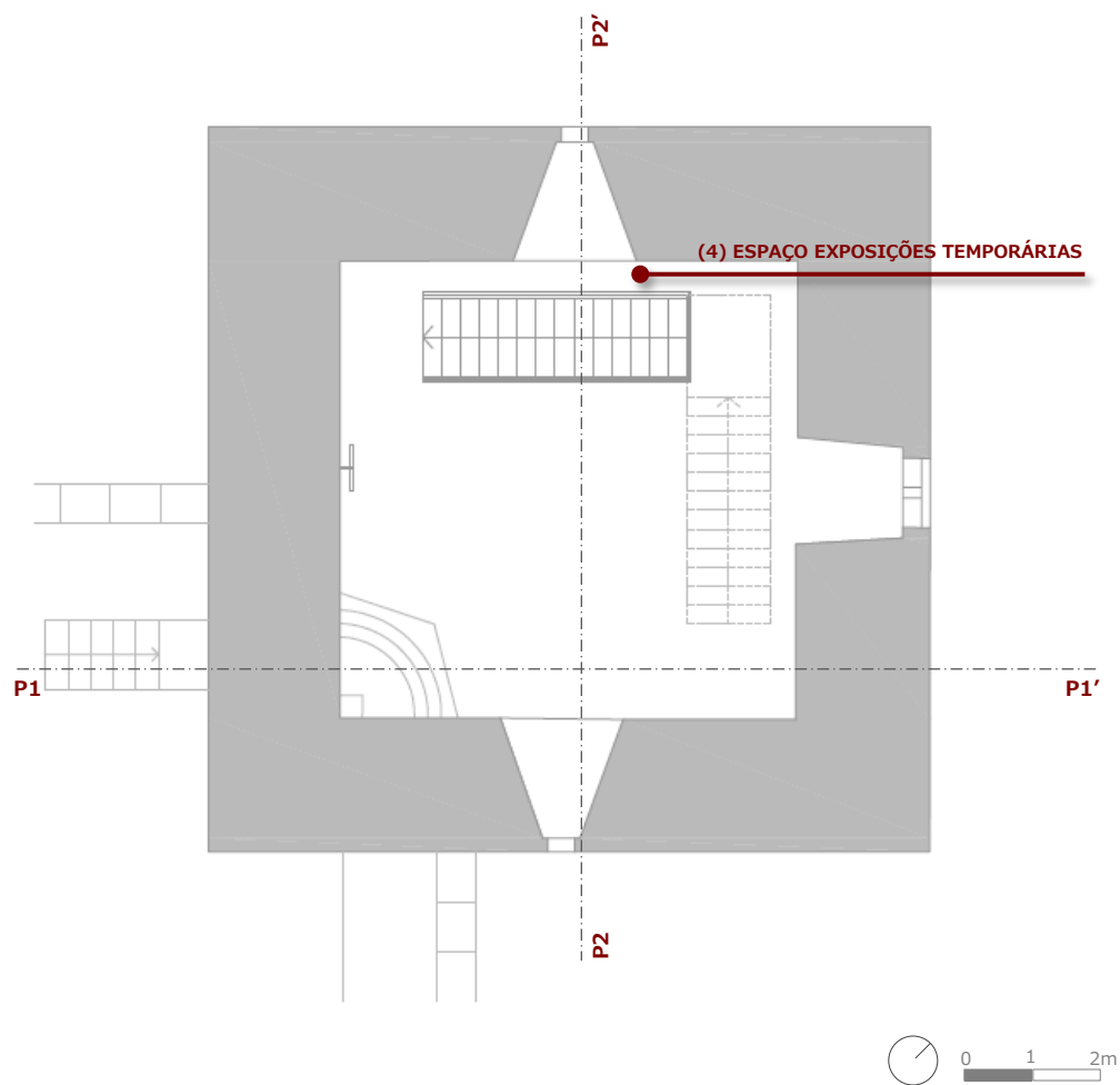
Figura 7.139. Planta do piso 4. Adaptado pela autora.
