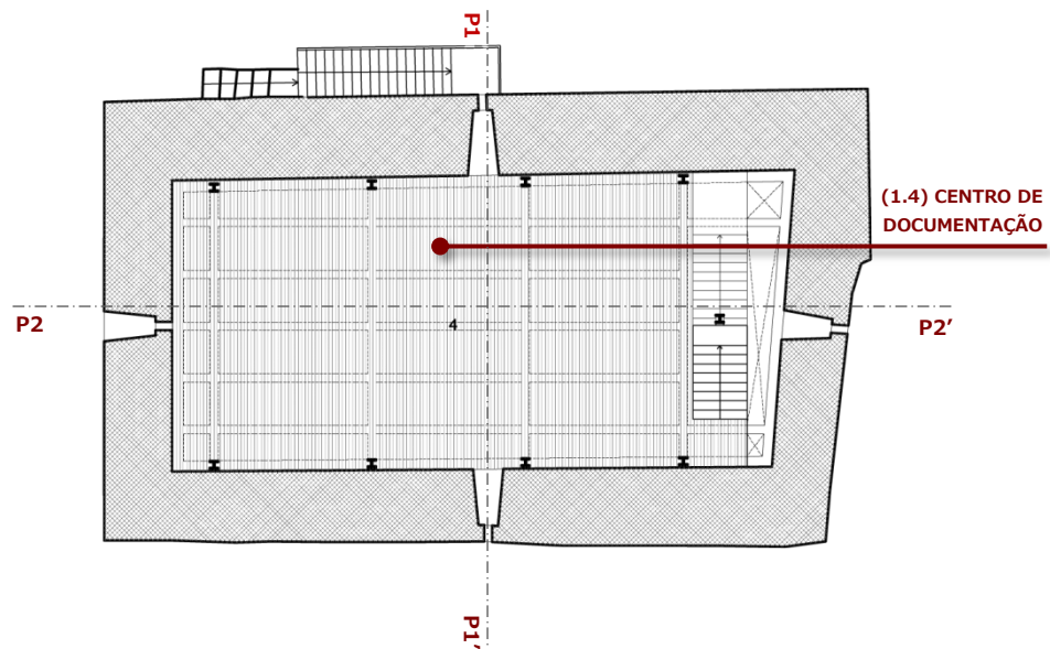
Figura 7.80. Planta do Piso 2. Adaptado pela autora.
