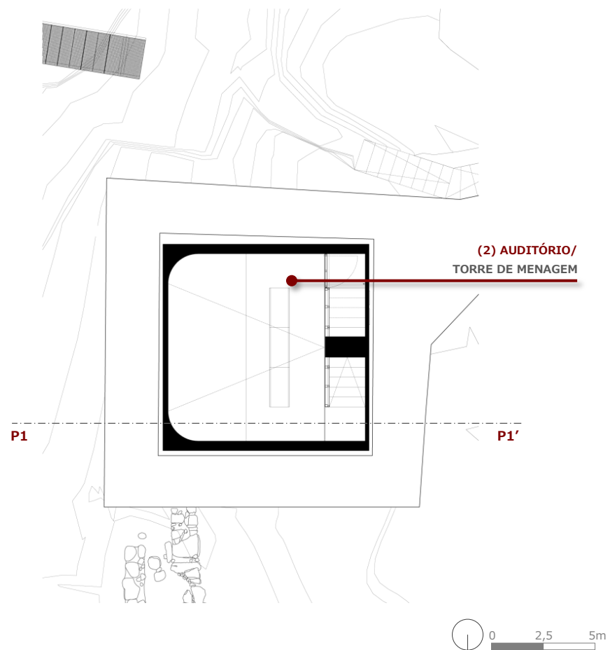
Figura 7.113. Planta inferior da sala de audiovisuais. Adaptado pela autora.
