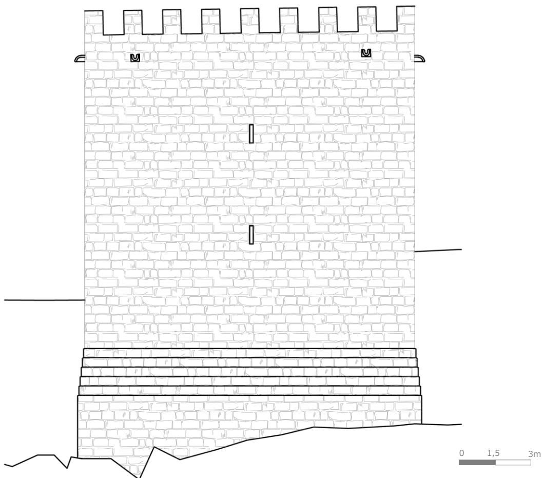
Alçado posterior.
