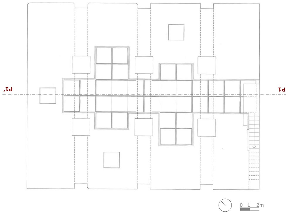
Planta da cisterna/algibe. Adaptado pela autora. (Ferreira, ed., 2009, 64).
