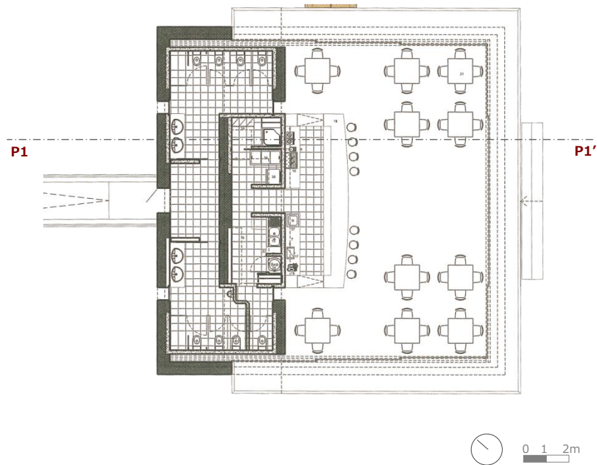
Figura 7.194. Planta da casa de chá. Adaptado pela autora.
