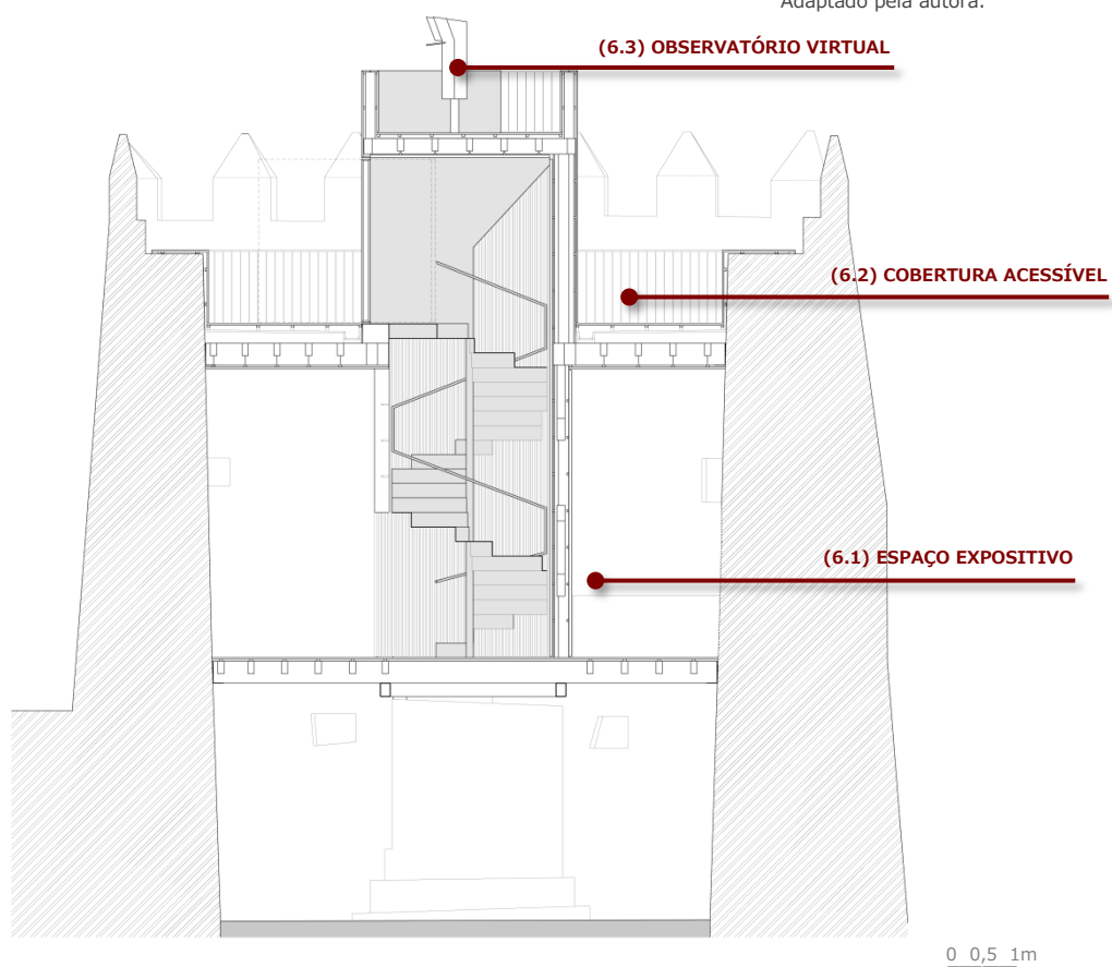
Figura 7.51. Perfil 1. Adaptado pela autora.
