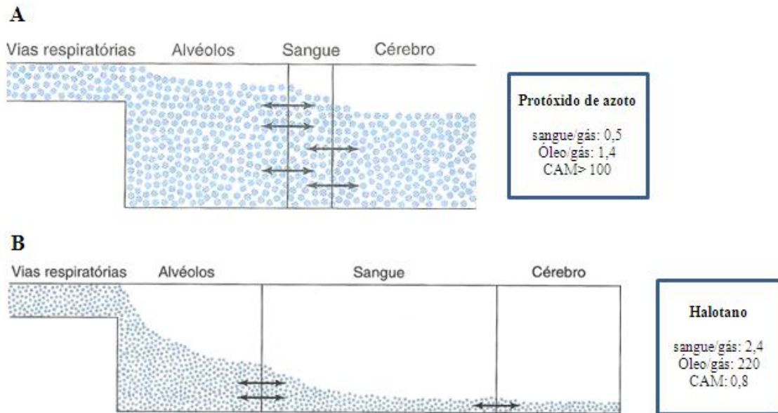
Figura 3 - Comparação da rapidez de indução do protóxido de azoto com o halotano. A solubilidade é representada pelo tamanho do compartimento, e o grau de preenchimento de cada um reflete a pressão parcial de cada anestésico. A: Protóxido de azoto tem baixa solubilidade no sangue e são necessárias menores moléculas para provocar uma alteração de pressão. B: Halotano com grande solubilidade no sangue e necessita de mais moléculas para alterar a pressão (Adaptado de: Katzung, 2008).
